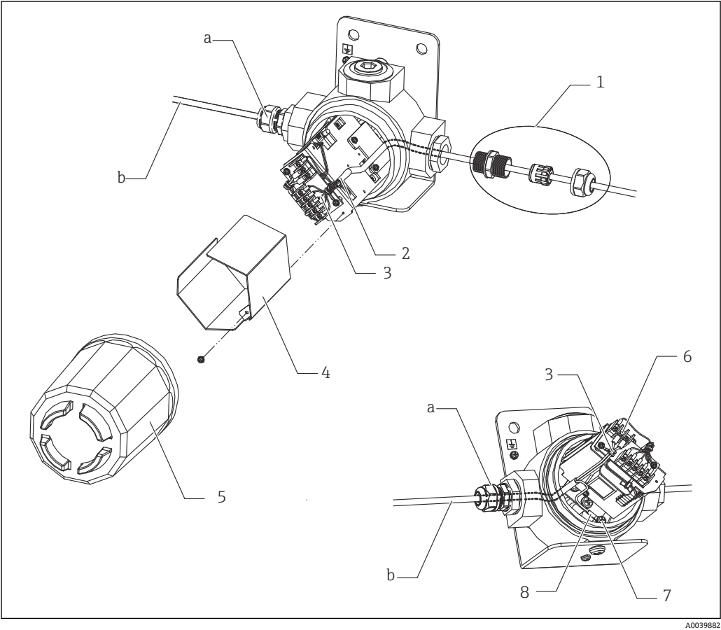
图 14 NAR300-x6xxxx 和防爆型传感器数据转换盒电缆安装示意图
