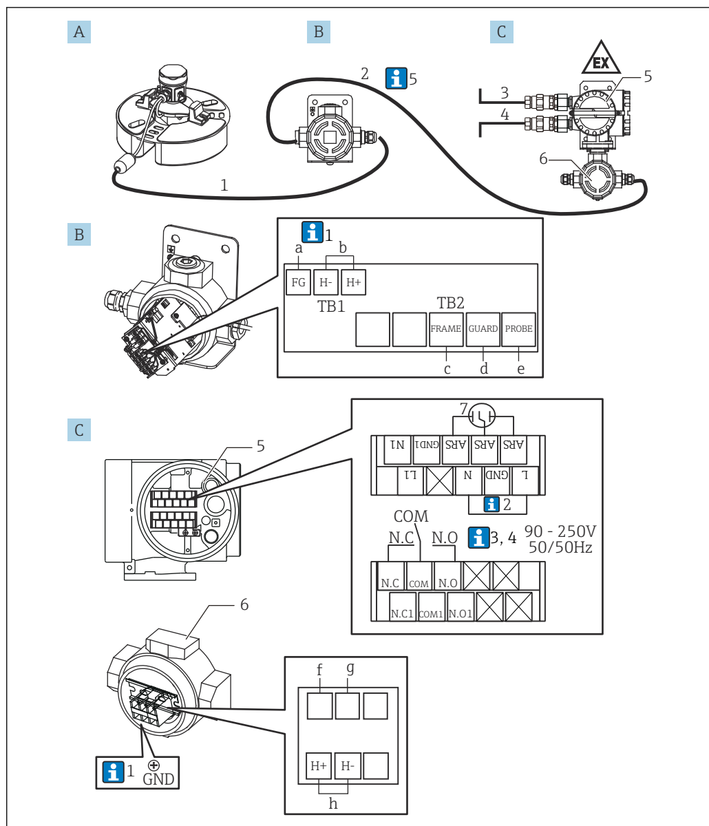
图 18 本安防爆型 (Ex d [ia]) 转换器 NRR261-5 接线示意图
