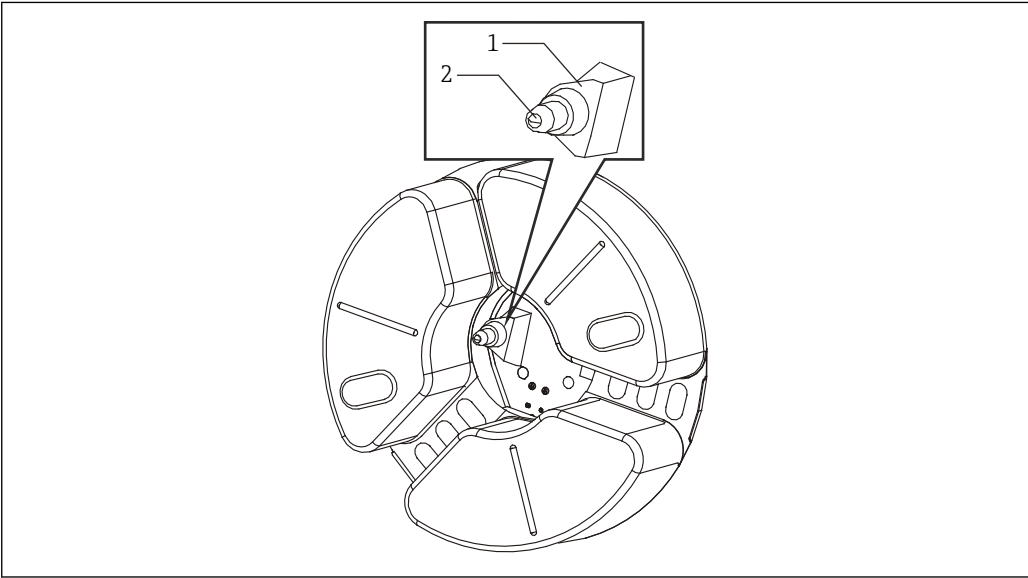
图 21 传感器清洁
