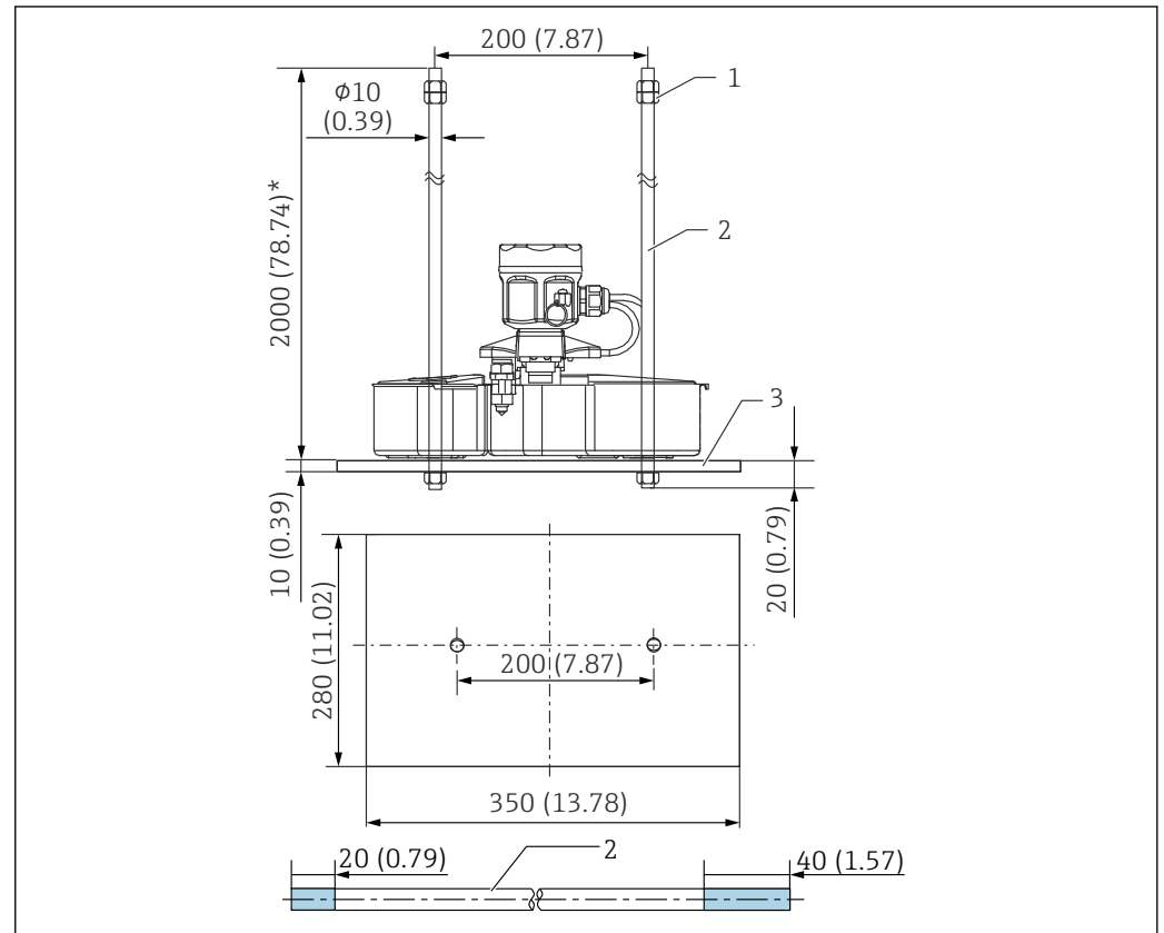
图 13 NAR300/浮子导杆
