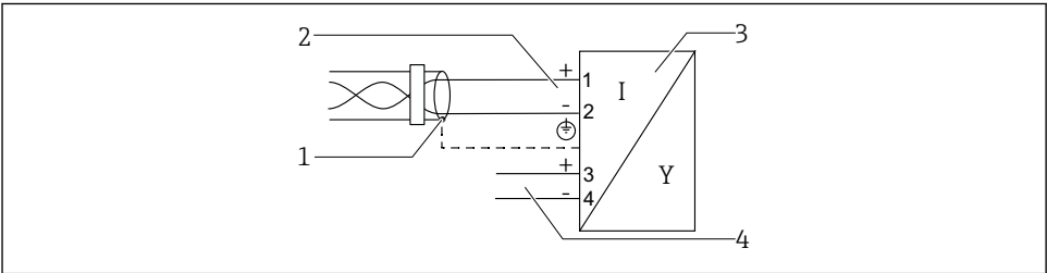
图 4 接线图: PROFIBUS PA / FOUNDATION Fieldbus
