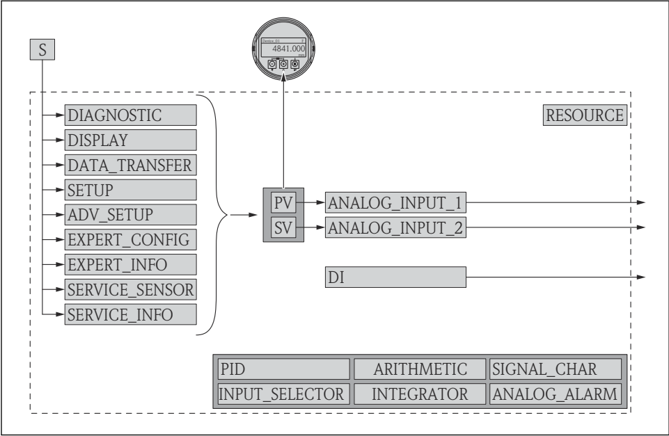
图 9 设备块的出厂设置
