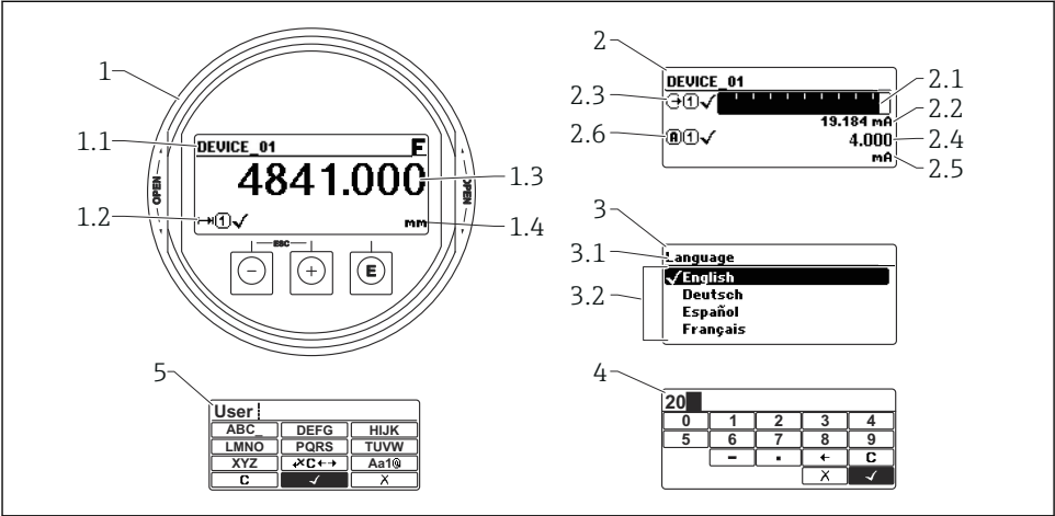
图 11 显示与操作单元的显示格式
