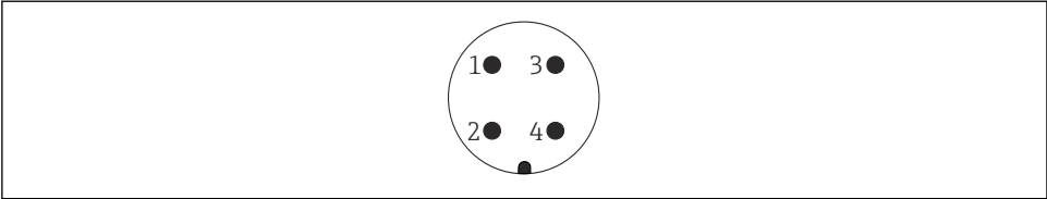
图 5 7/8"插头的针脚分配
