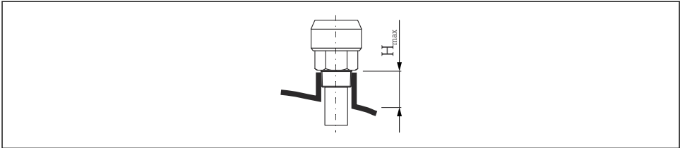
图 2 全密封喇叭天线（FMR50）的安装短管高度示意图； H_{\max} = 60 \text{ mm} (2.36 in)
