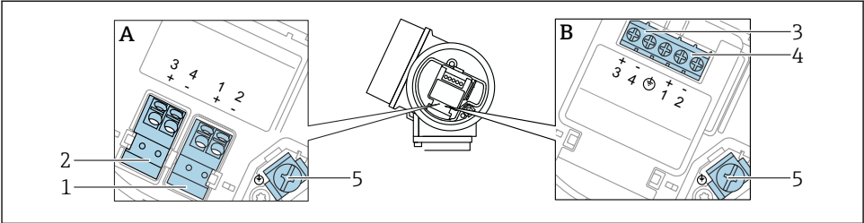
图 3 接线端子分配 PROFIBUS PA / FOUNDATION Fieldbus
