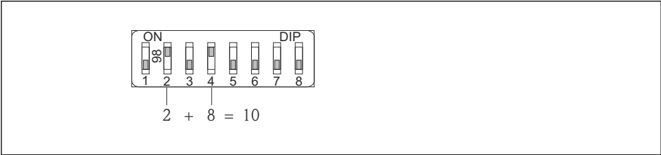
图 9 硬件地址设定实例；开关 8 拨至“OFF”位置；开关 1...7 确定设备地址。
