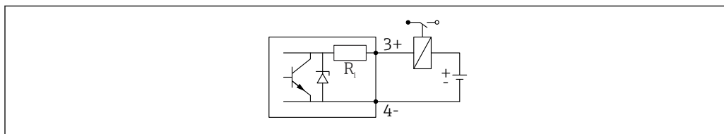
17 Подключение реле
