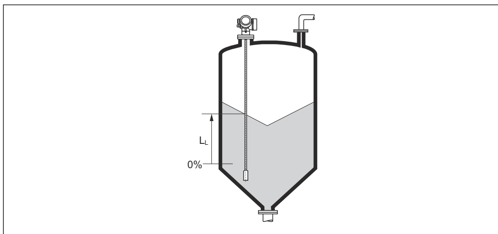
38 Уровень при измерении в сыпучих средах
