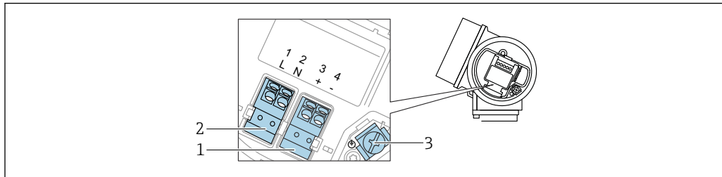
14 Назначение клемм, 4-проводное подключение: 4 до 20 мА HART (90 до 253 В AC )
