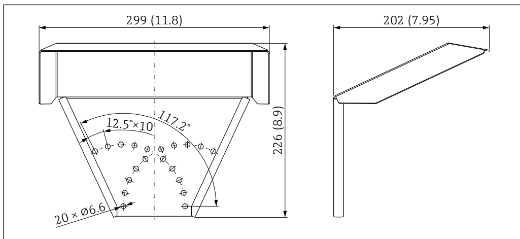
33 Размеры. Единица измерения мм (дюйм)
