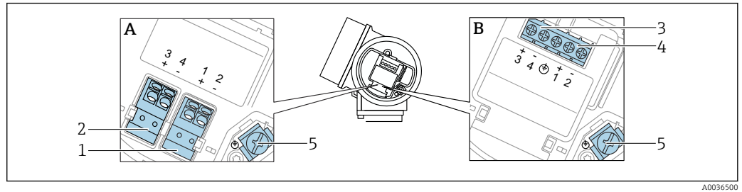
15 Назначение клемм; PROFIBUS PA/FOUNDATION Fieldbus
