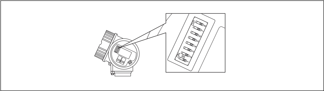
24 Переключатель адресов в клеммном отсеке
