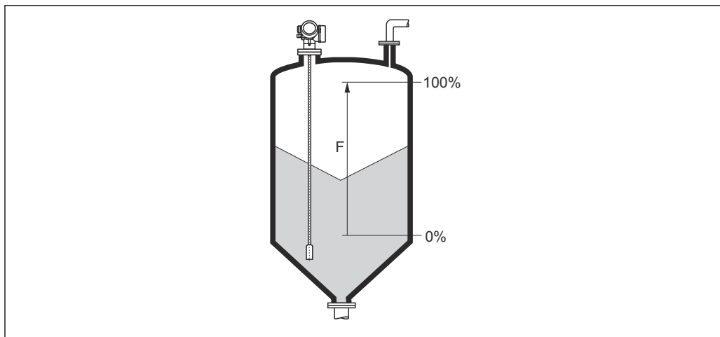
37 Калибровка полной емкости (F) для измерения уровня сыпучих сред
