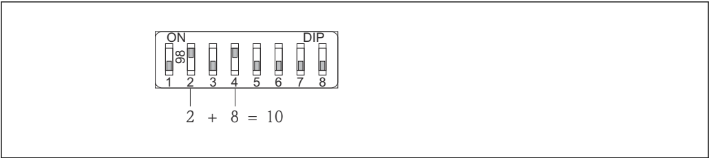
25 Пример аппаратной адресации: переключатель № 8 переведен в положение OFF; переключатели №№ 1–7 определяют адрес.
