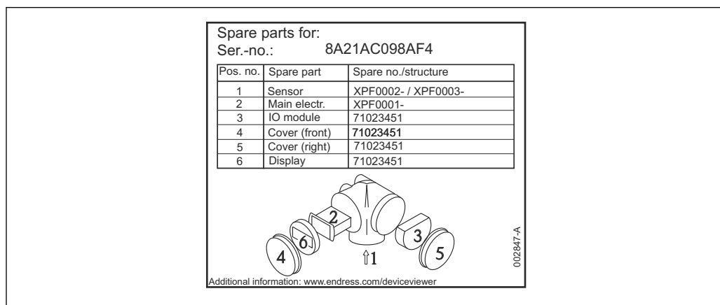
31 Пример заводской таблички с перечнем запасных частей, размещаемой на крышке присоединительного отсека
