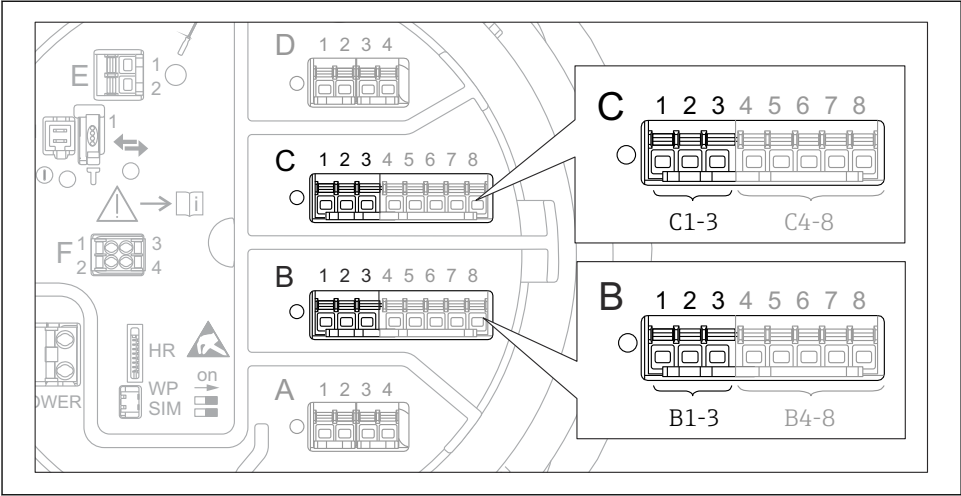
图 22 用作 4...20 mA 输入的模拟量输入/输出模块的安装位置示意图。设备的订货号确定当前使用的模块。
