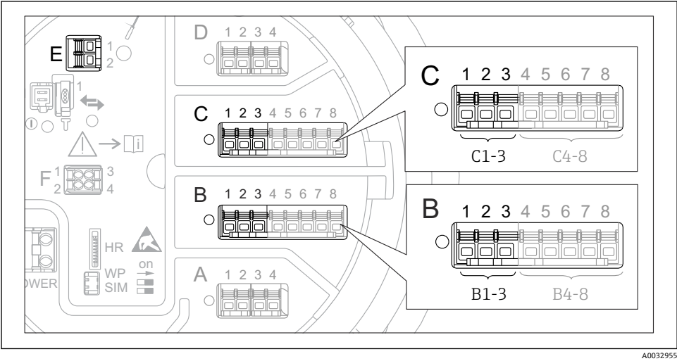
图 21 HART 回路的可能接线端子
