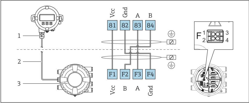
图 7 分离型显示单元与操作单元 DKX001 连接至罐旁指示仪 (NMR8x、NMS8x 或 NRF8x)
