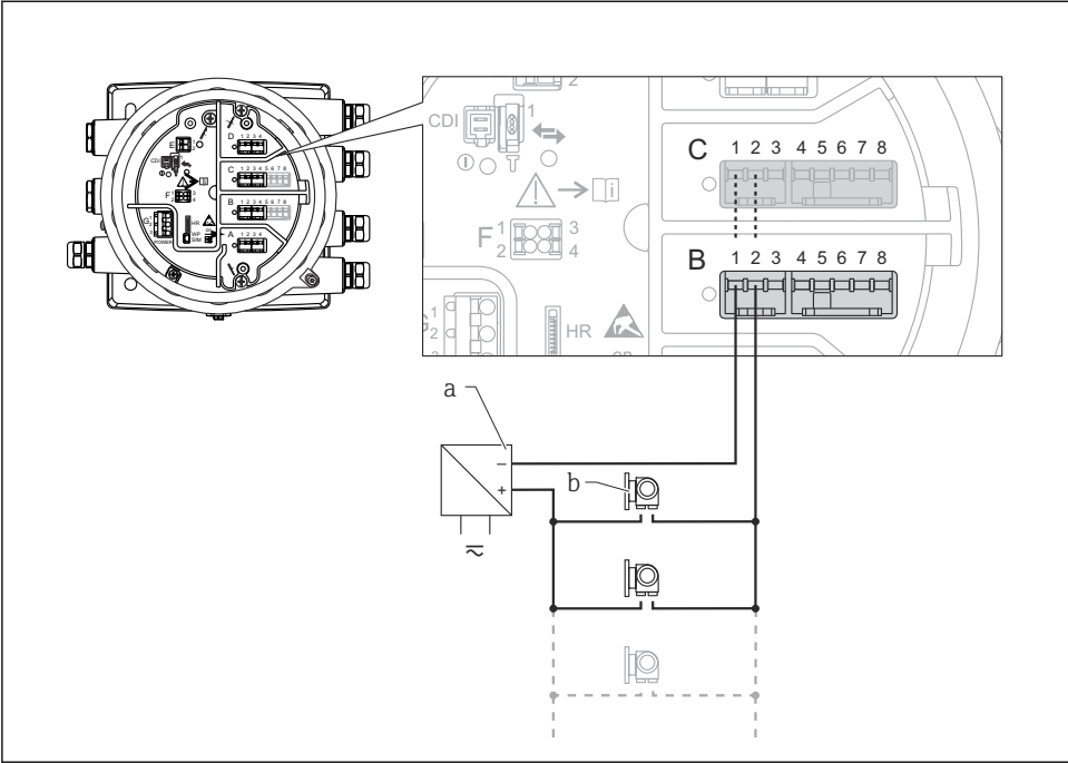
11 HART 主站模式下的无源模拟量输入/输出模块
