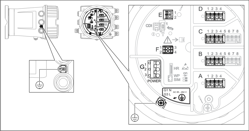
5 端子接线腔（典型实例）和接地端子示意图
