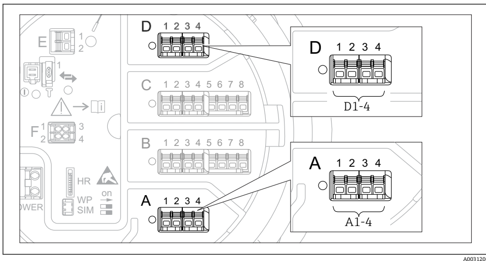
图 28 Modbus 模块或 V1 模块的安装位置示意图；取决于设备版本号，上述模块也可以安装在插槽 B 或 C 中。
