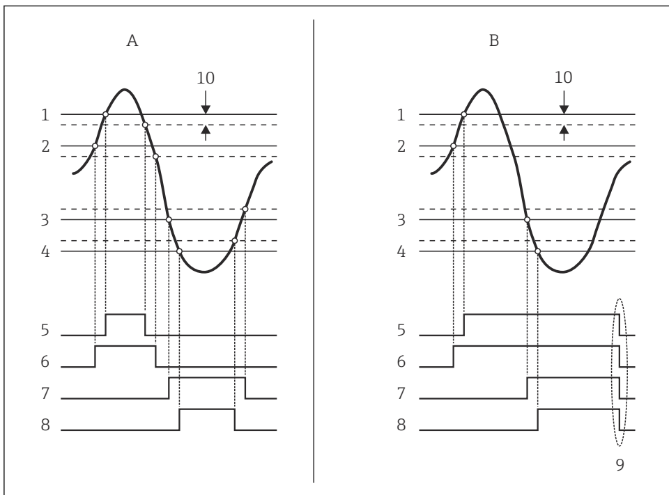
图 26 限定值计算原理
