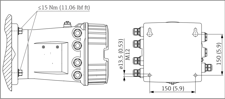
图 2 罐旁指示仪的墙装示意图
