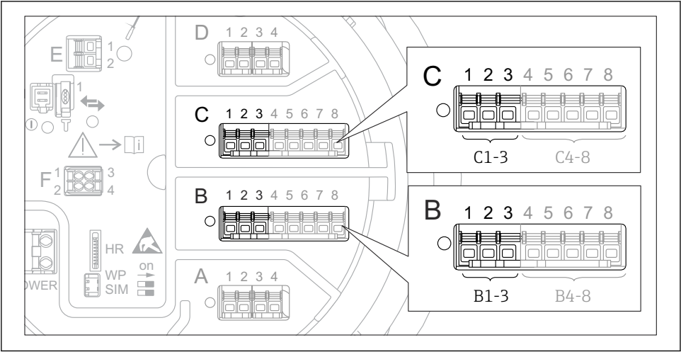
图 27 用作模拟量输出的模拟量输入/输出模块的安装位置示意图。设备的订货号确定当前使用的模块。
