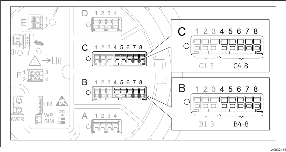
图 24 已连接 RTD 的模拟量输入/输出模块的安装位置示意图。设备的订货号确定当前使用的模块。
