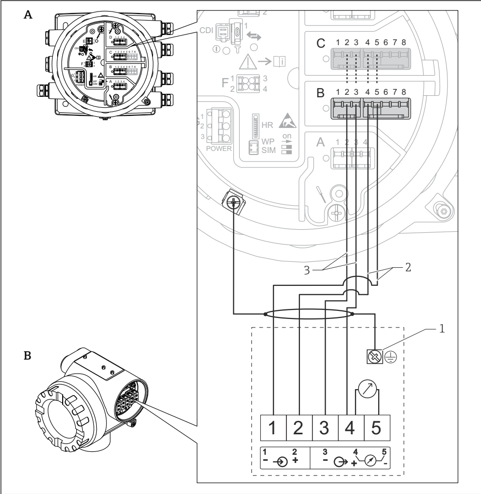
15 将 Micropilot S FMR5xx 连接至 Tankside Monitor NRF81 的模拟量输入模块
