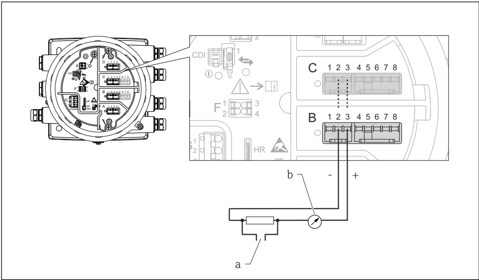
图 12 输出模式下的有源模拟量输入/输出模块
