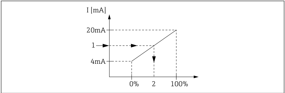
23 4...20 mA 输入对应过程变量
