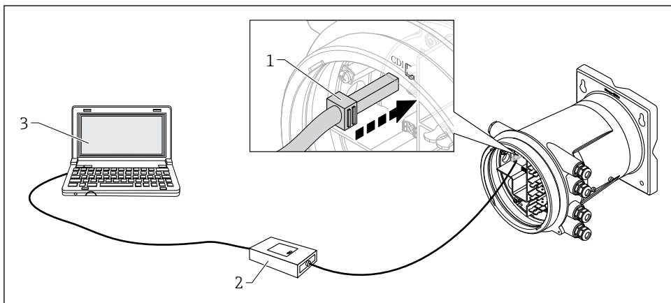
图 20 通过服务接口操作
