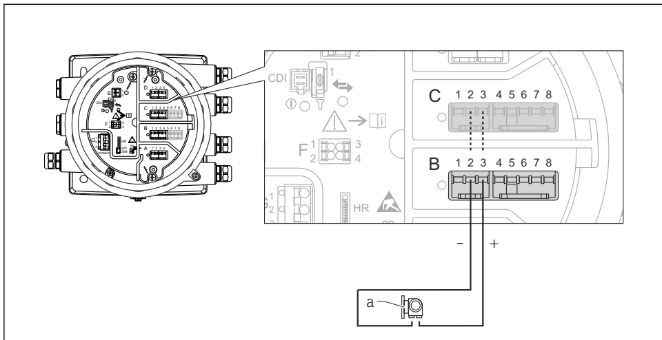
图 13 输入模式下的有源模拟量输入/输出模块
