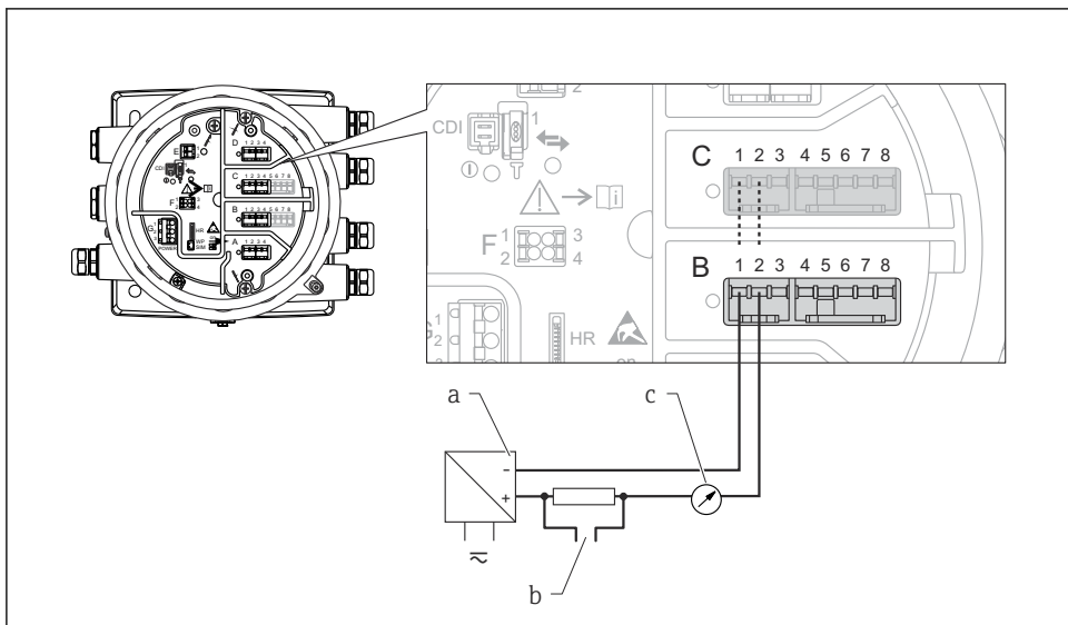
图 9 输出模式下的无源模拟量输入/输出模块
