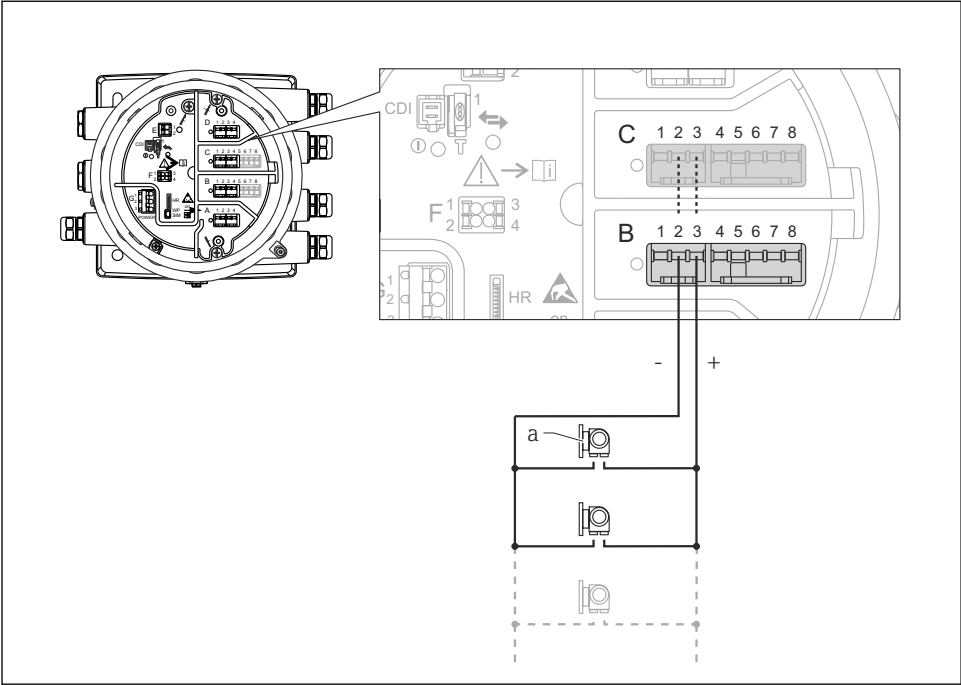
14 HART 主站模式下的有源模拟量输入/输出模块
