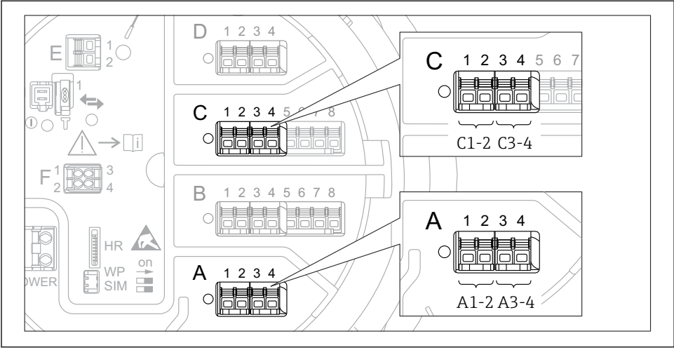
图 25 数字量输入/输出模块的可能安装位置（示例）；订货号确定数字量输入模块的数量和位置。
