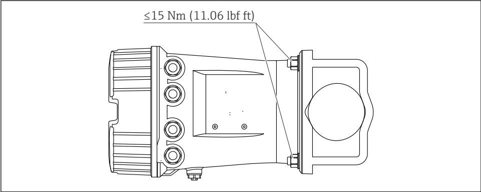
4 在水平管道中安装罐旁指示仪
