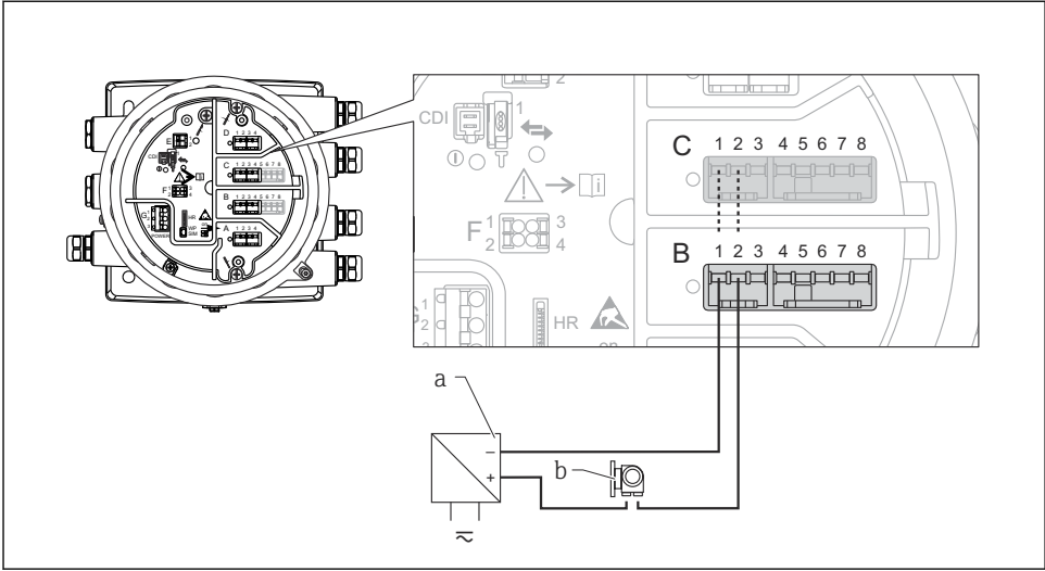
图 10 输入模式下的无源模拟量输入/输出模块
