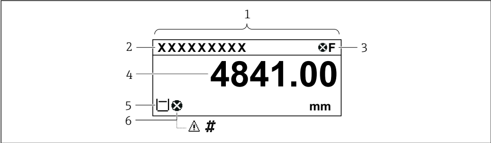
图 18 典型的标准显示界面（测量值显示）
