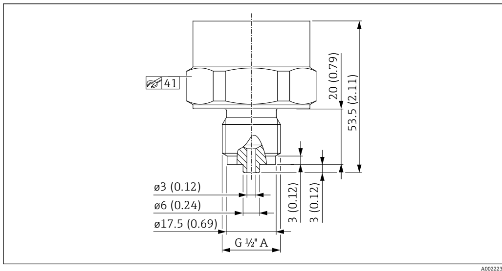
图 5 ISO 228 G 1/2" A 螺纹, EN 837。测量单位 mm (in)
