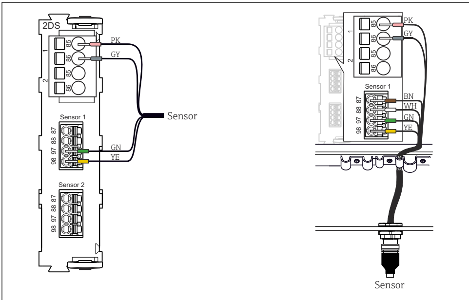
16 Sensoraansluiting op de sensoringang (links) of via M12-connector (rechts)
