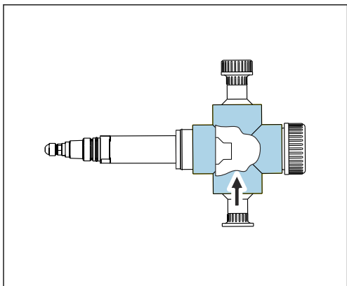
13 Installeren met CYA251 doorstroomarmatuur
