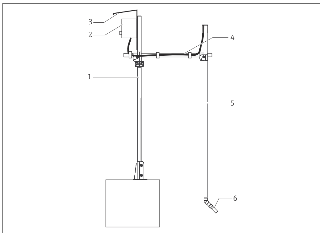
10 Sistema di misura con armatura di immersione (esempio)
