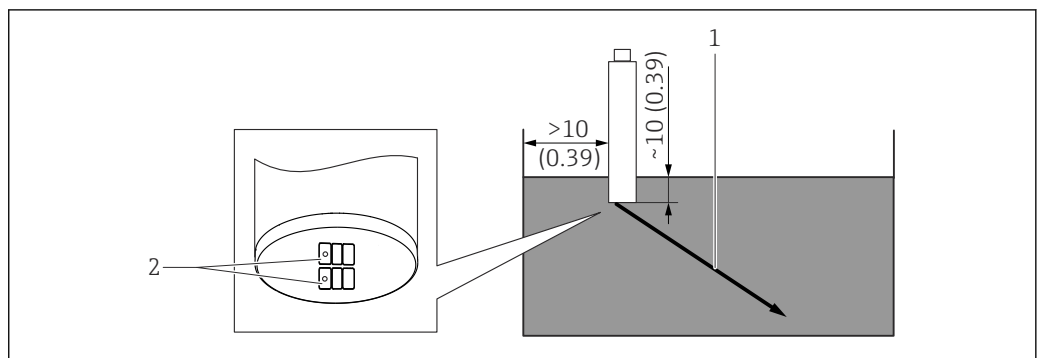
34 Posizionamento del sensore. Dimensioni: mm (in)
