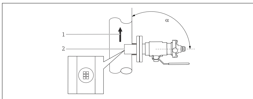
13 Installazione con armatura retrattile
