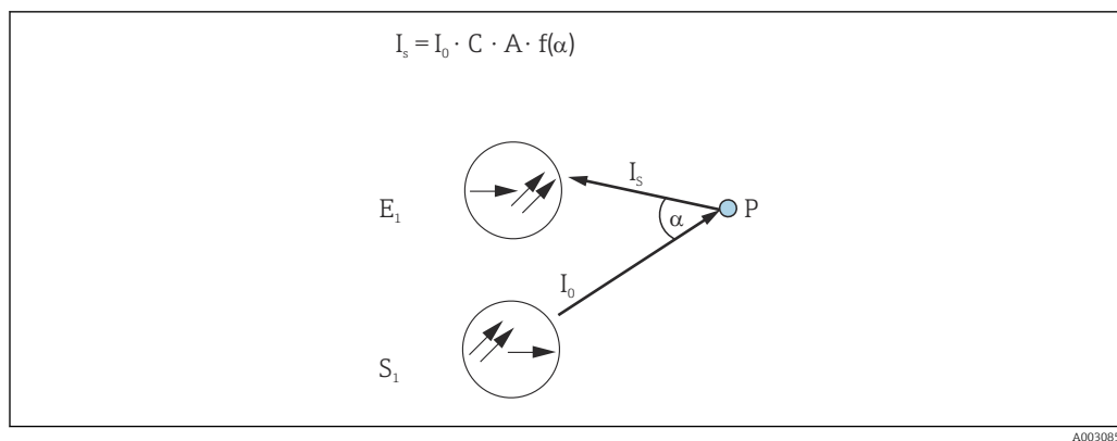
7 Principio del metodo di back scattering
