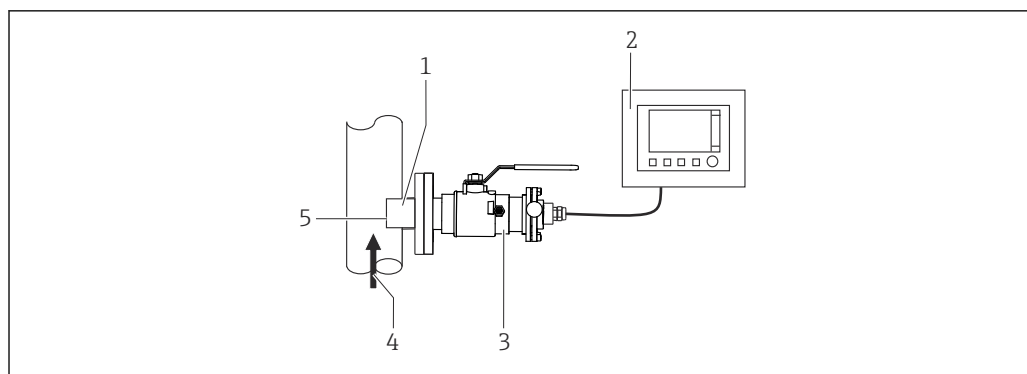
12 Sistema di misura con armatura retrattile (esempio)
