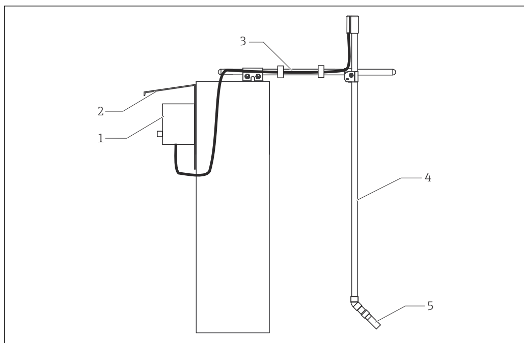
11 Sistema di misura con armatura di immersione (esempio)
