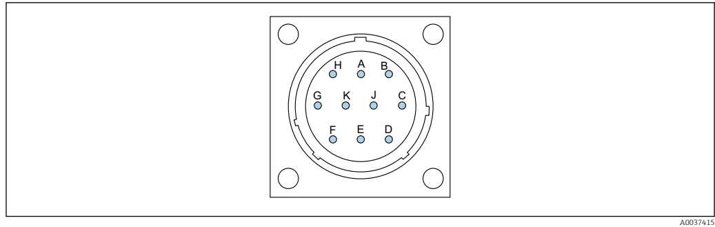
■ 15 Asignación de terminales del conector de 10 patillas
