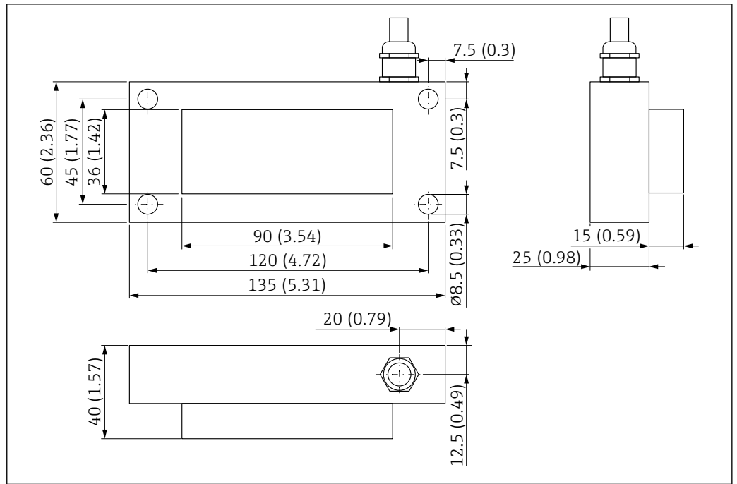
8 Medidas. Unidad de medida mm (in)
