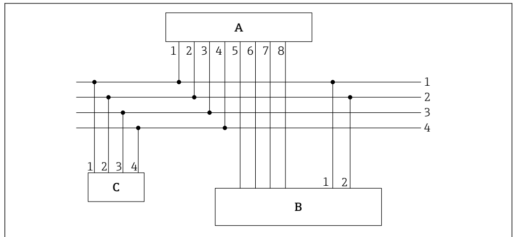
19 Ejemplo de conexión, cable con toma de 10 pines (en el lateral del equipo) y terminales de empalme en los extremos del cable
