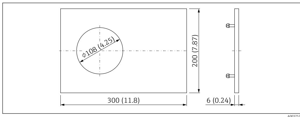
24 Placa deflectora, 1.4301, escotadura para el sensor de \varnothing 108 mm (4,25 in). Unidad de medida mm (in)
