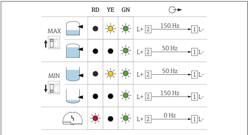
24 Schaltverhalten und Signalisierung, Elektronikeinsatz FEL67
