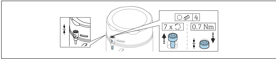
5 Deckel mit Sicherungsschraube; Hygienegehäuse (nur bei Staubexplosionsschutz)
