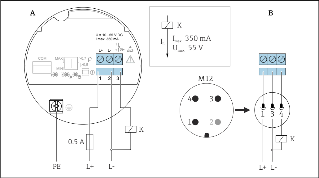
19 3-Leiter DC-PNP, Elektronikeinsatz FEL62 A Anschlussverdrahtung mit Klemmen B Anschlussverdrahtung mit Stecker M12 im Gehäuse gemäß Standard EN61131-2
