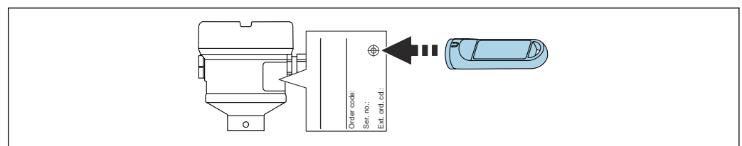
41 Funktionstest mit Testmagnet
