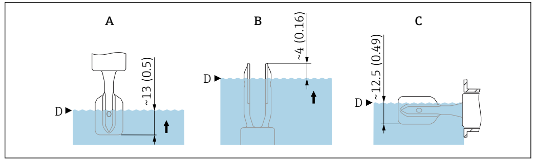
4 Typische Schalterpunkte. Maßeinheit mm (in)
