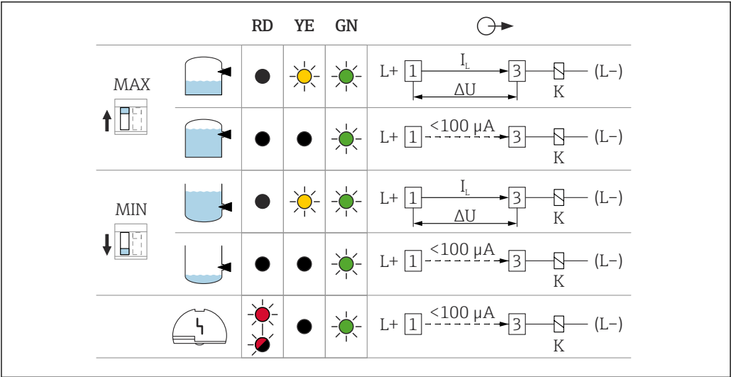
20 Verhalten Schaltausgang und Signalisierung, Elektronikeinsatz FEL62 MAXDIP-Schalter, MAX-Sicherheit einstellen MIN DIP-Schalter, MIN-Sicherheit einstellen RD LED rot für Warnung oder Alarm YE LED gelb Schaltzustand GN LED grün Betriebszustand, Gerät ein I_L Laststrom durchgeschaltet
