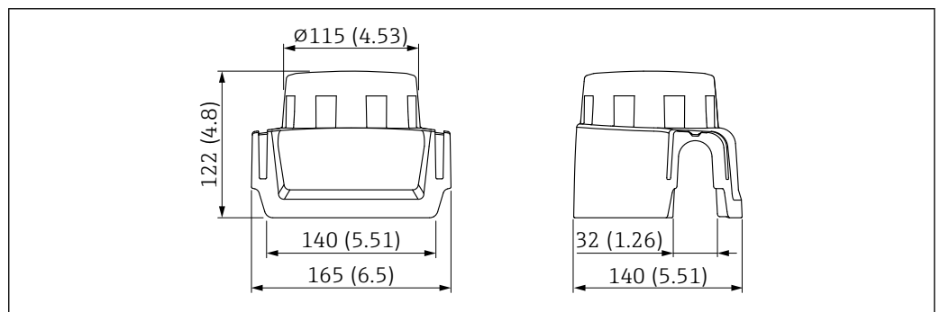
45 Wettergeschutzhäube für Einkammer Gehäuse Aluminium oder 316L. Maßeinheit mm (in)
