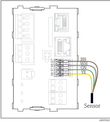
30 Memosens-Sensoren ohne zusätzliche Versorgungsspannung
