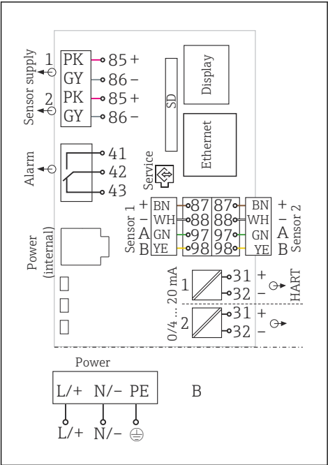
25 Gesamt-Anschlussplan am Beispiel BASE2-E und Erweiterungsnetzteil (B)
