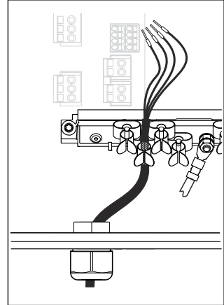
23 Kabel in Erdungsschelle eindrücken
