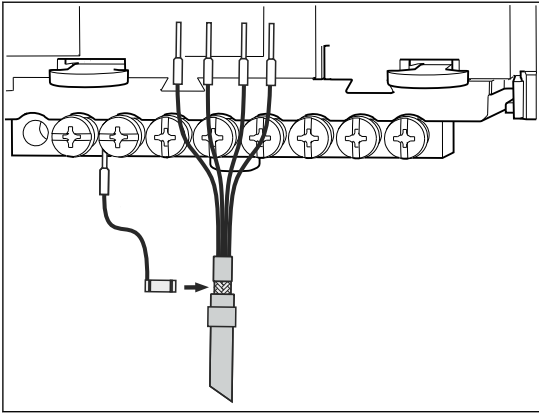
29 Funktionserdanschluss
