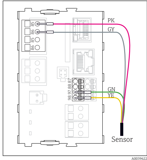
31 Memosens-Sensoren mit zusätzlicher Versorgungsspannung
