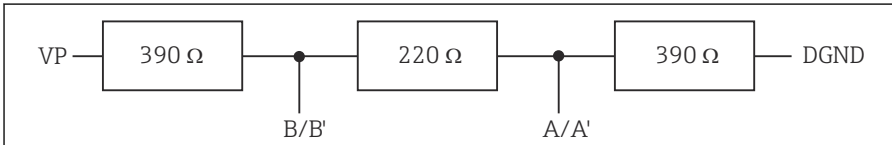
62 Aufbau der internen Terminierung
