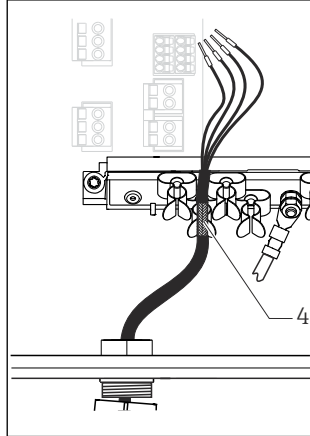
22 Kabel auf Erdungsschelle auflegen
