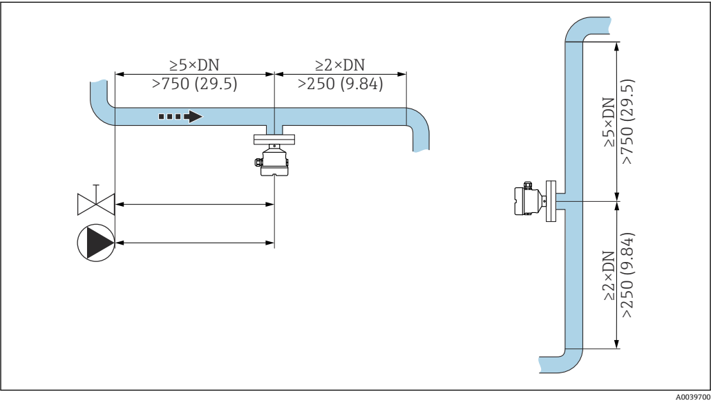
图 7 前直管段的安装。测量单位 mm (in)
