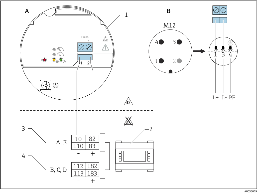
图 17 电子插件 FEL60D 和密度计算仪 FML621 的接线图
