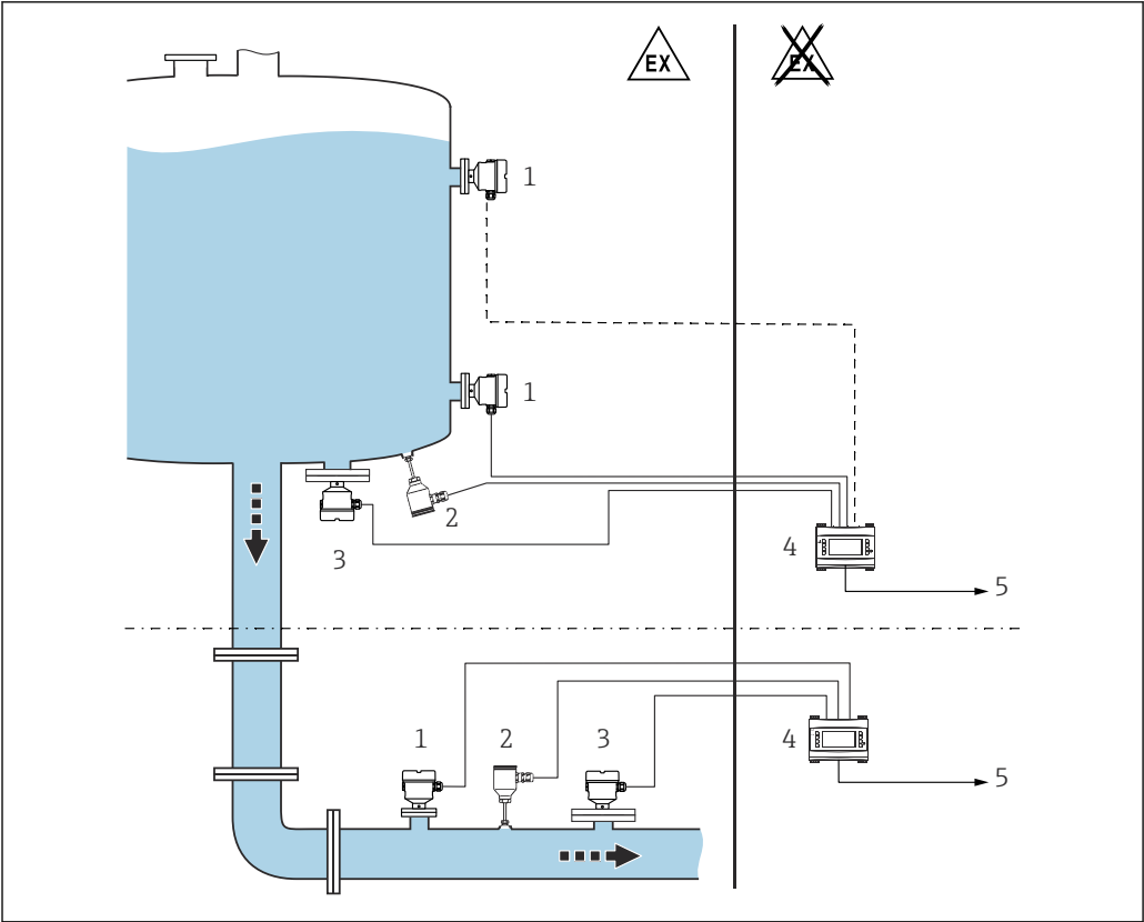
图 18 与密度计算仪 FML621 配套进行密度测量
