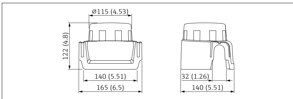
图 22 保护盖，适用单腔体铝外壳或 316L 外壳。测量单位 mm (in)
