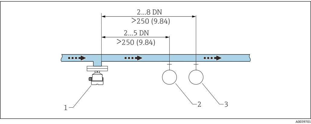
图 8 后直管段的安装。测量单位 mm (in)
