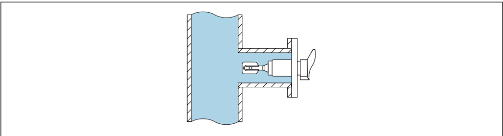
图 6 安装实例: 叉体不接触管道内流动的介质
