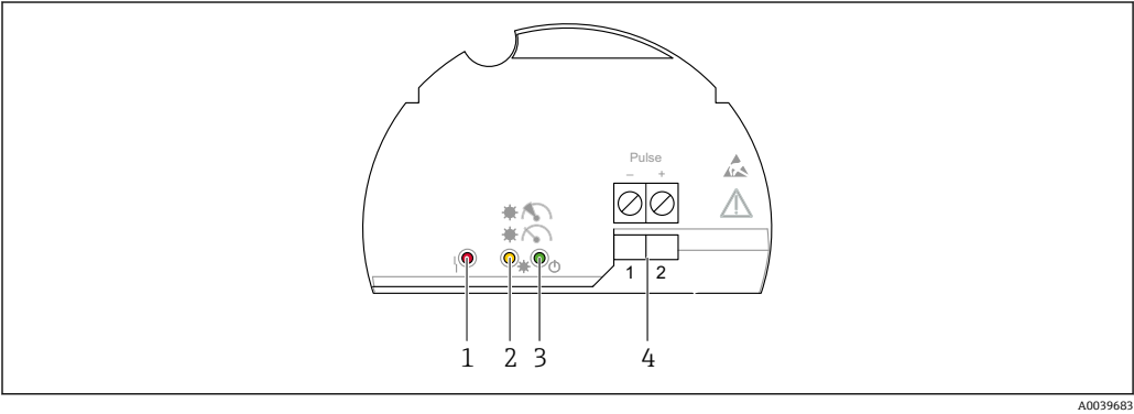
图 20 电子插件 FEL60D
