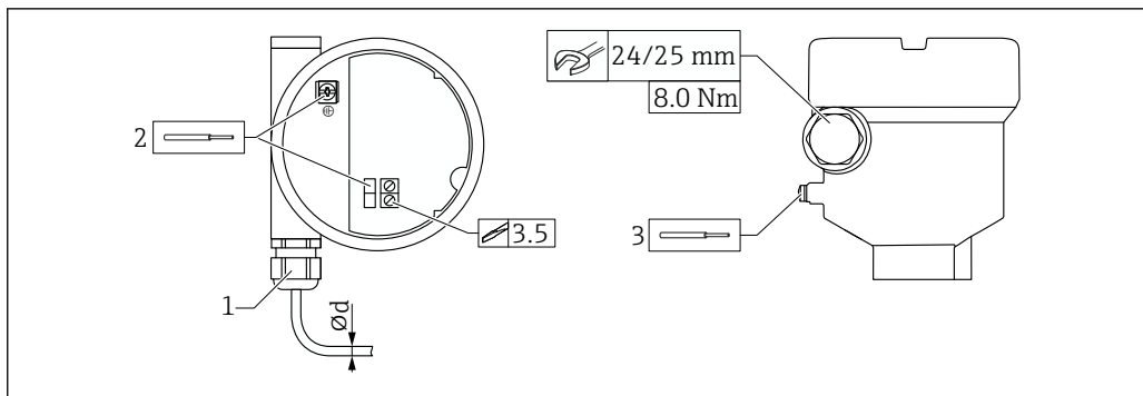
图 19 实例：接头（带电缆入口）和电子插件（带接线端子）
