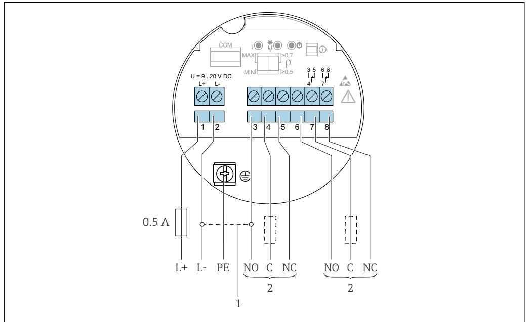
图 25 电子插件 FEL64 DC: 直流连接型, 带继电器输出
