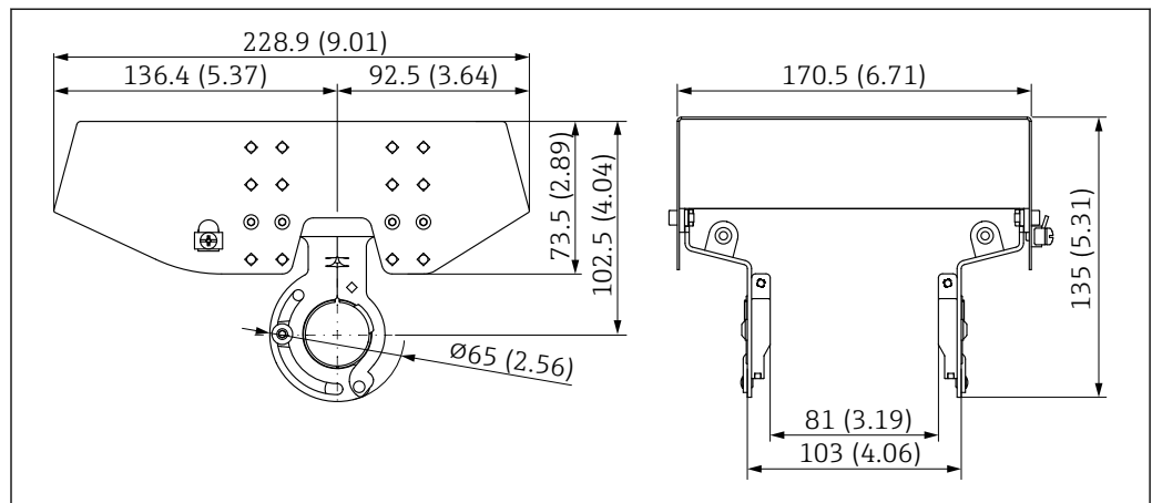
图 47 双腔体铝外壳的防护罩。测量单位 mm (in)
