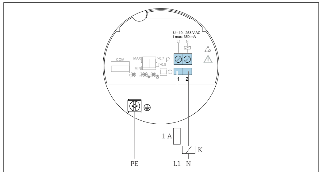
图 18 FEL61 电子插件: 两线制连接, 交流 AC 型
