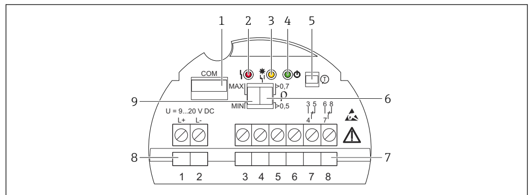
图 34 实例：电子插件 FEL64DC
