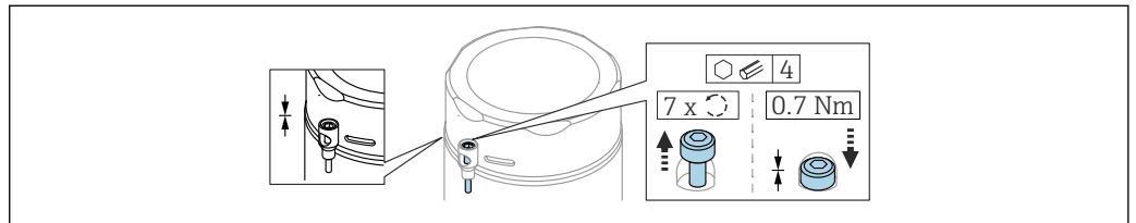
图 17 带锁定螺丝的外壳盖；卫生型外壳（仅适用粉尘防爆场合）
