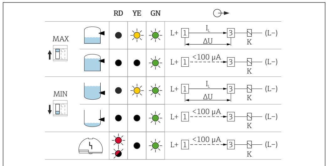
图 22 电子插件 FEL62 的继电器响应和故障信号
