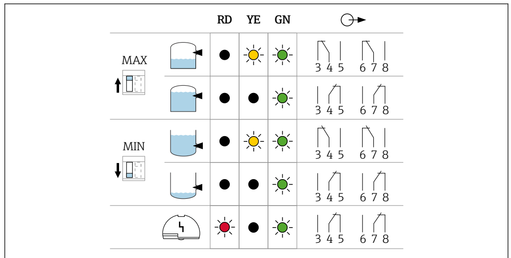
图 24 电子插件 FEL64 的继电器响应和故障信号
