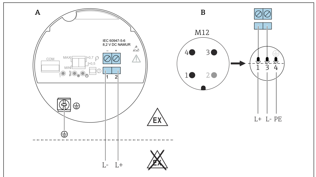
图 29 电子插件 FEL68: 两线制连接, NAMUR 信号 ( \geq 2.2 \text{ mA} / \leq 1.0 \text{ mA} )
