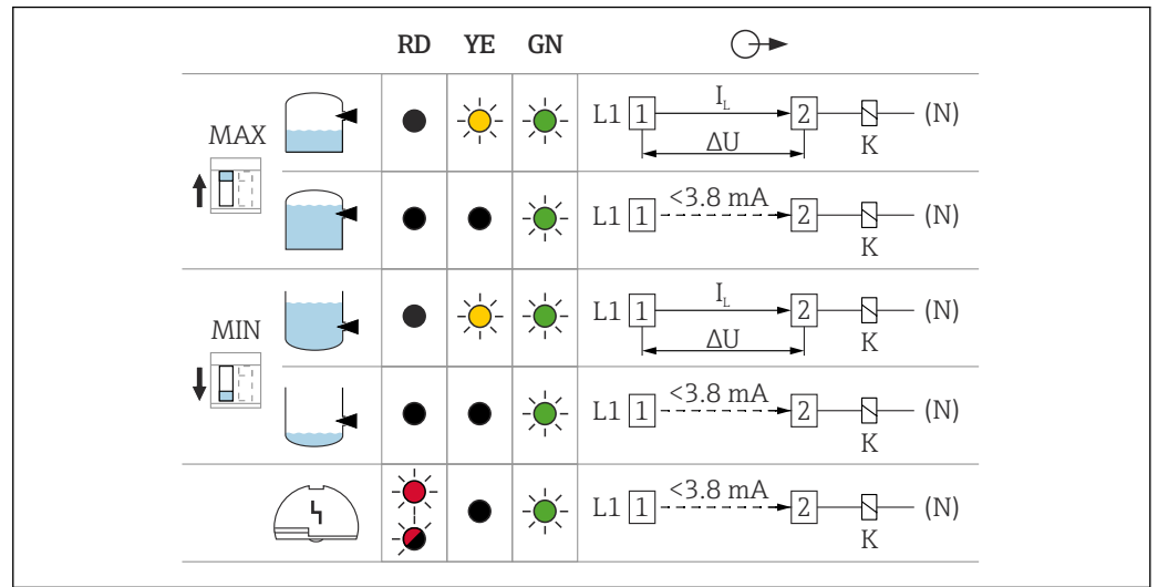
图 19 电子插件 FEL61 的继电器响应和故障信号
