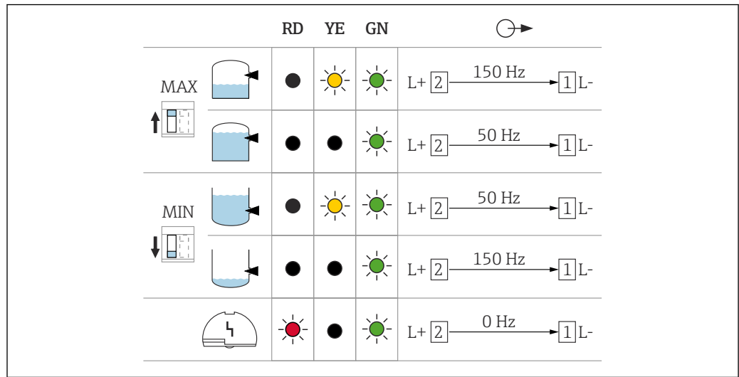
图 28 电子插件 FEL67 的继电器响应和故障信号
