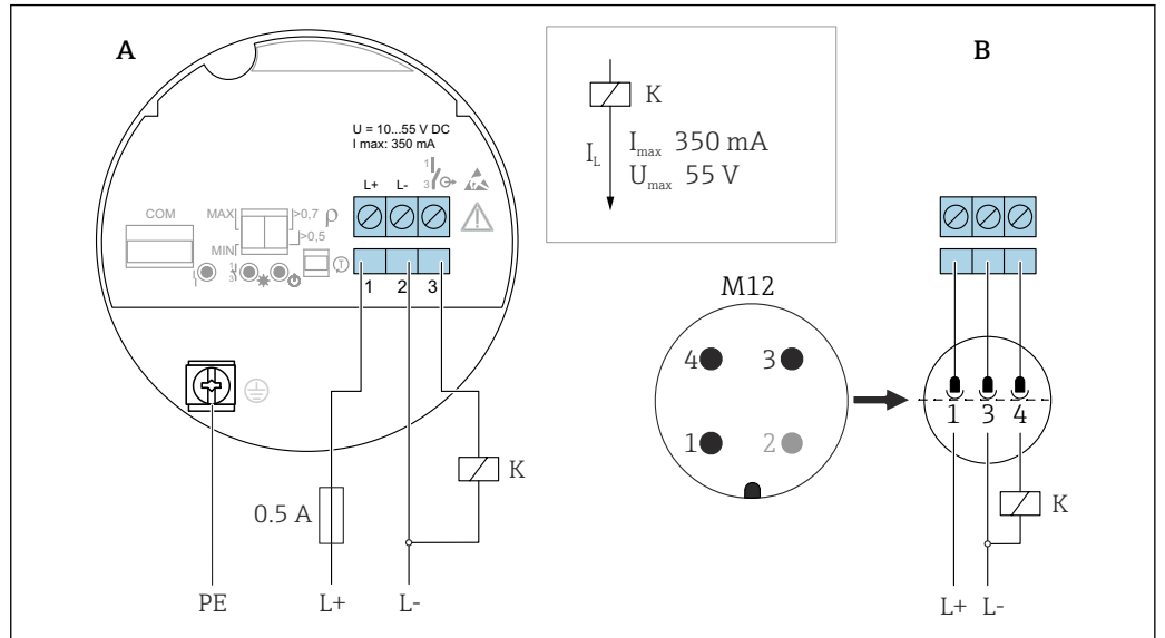
图 21 电子插件 FEL62: 三线制连接, 直流 DC-PNP 型
