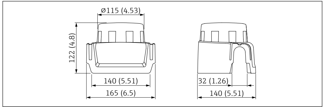
图 48 防护罩，适用单腔体铝外壳。测量单位 mm (in)
