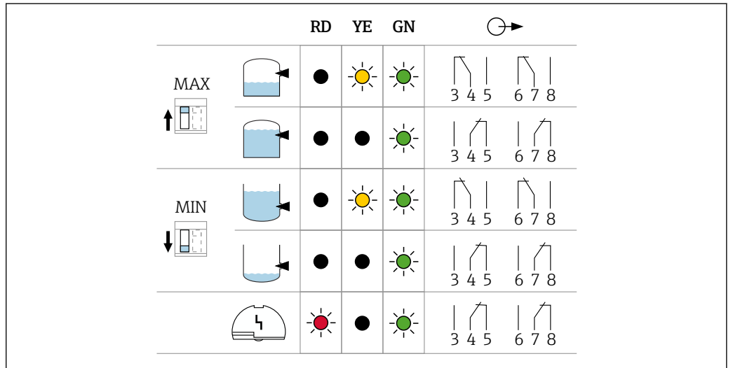
图 26 电子插件 FEL64 DC 的继电器响应和故障信号
