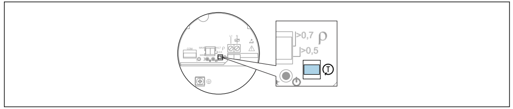
34 Tecla para la prueba de funcionamiento (módulos del sistema electrónico FEL61/62/64/64DC/67/68)
