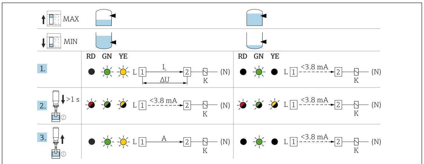
35 FEL61 comportamiento de la conmutación y señalización
