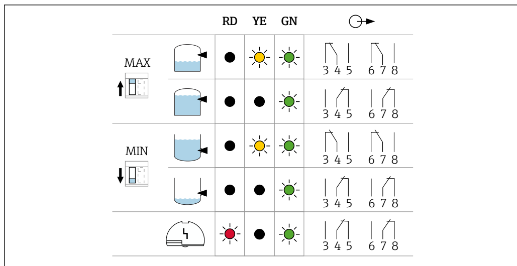
22 Comportamiento de la salida de conmutación y señalización, módulo de la electrónica FEL64
