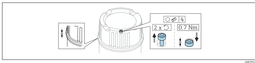
15 Tapa con tornillo de fijación
