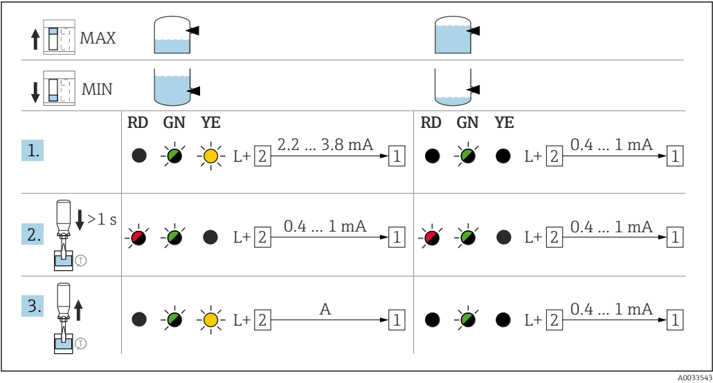
40 Comportamiento de conmutación y señales de la electrónica NAMUR
