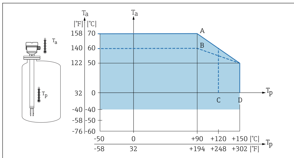
49 Temperatura ambiente admisible T_a en la caja en función de la temperatura de proceso T_p en el depósito:
