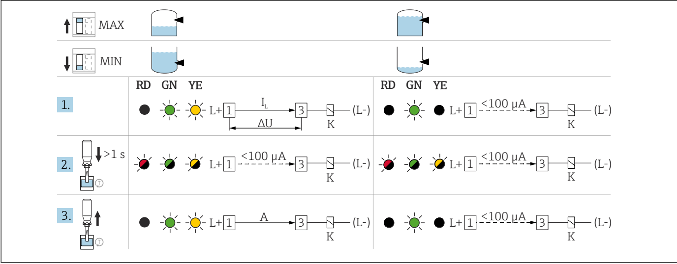
37 FEL62 comportamiento de la conmutación y señalización
