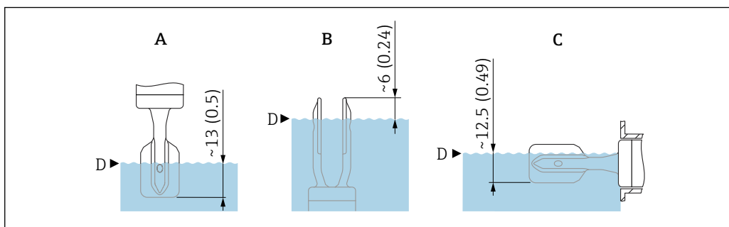
5 Puntos de conmutación típicos, diapasón recubierto de plástico (ECTFE, PFA). Unidad de medida mm (in)
