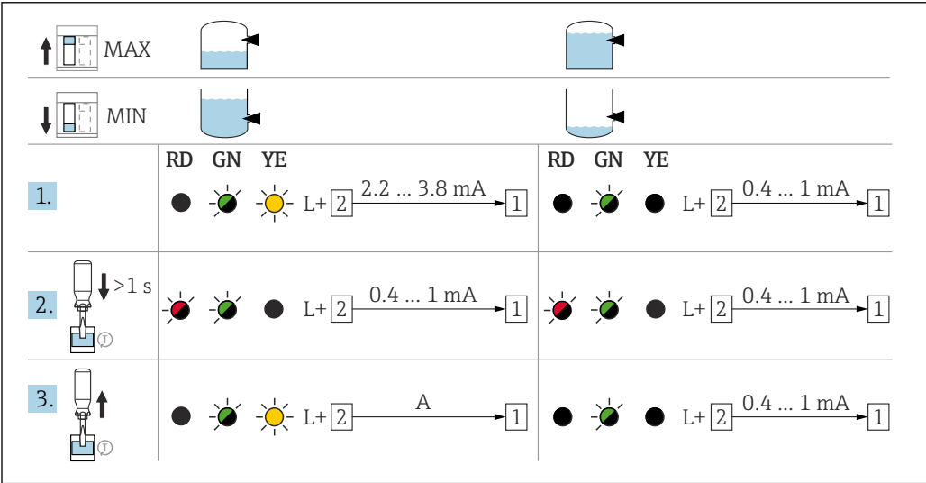
41 Comportamiento de conmutación y señales de la electrónica NAMUR
