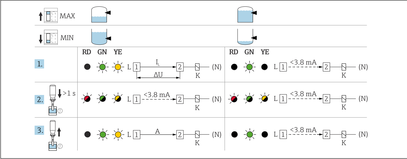
36 FEL61 comportamiento de la conmutación y señalización
