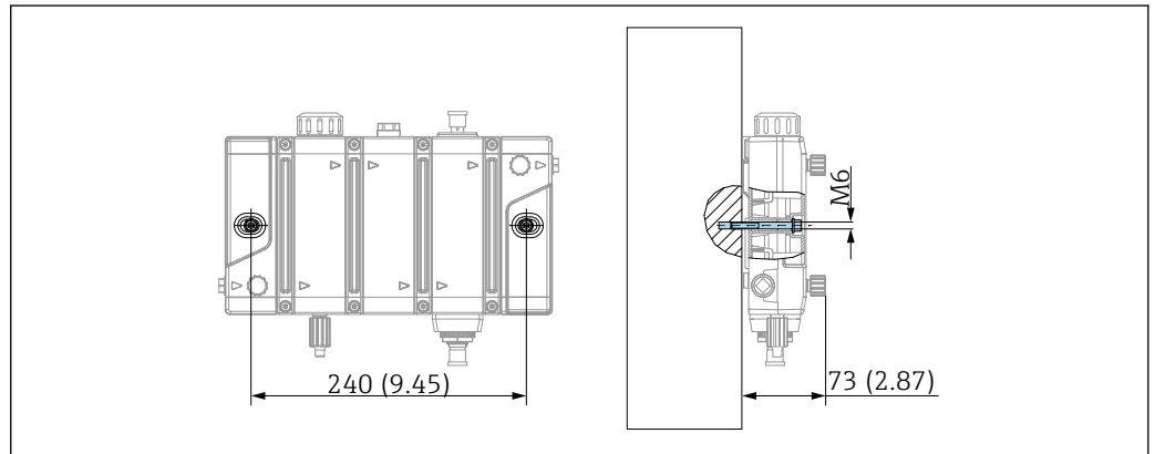
4 Montaggio direttamente a parete. Unità ingegneristica: mm (in)
