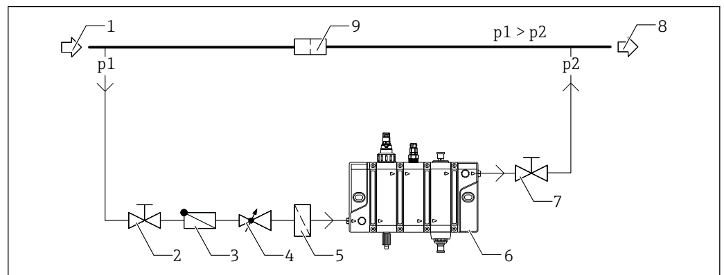
9 Esempio di connessione con bypass e orifizio nel tubo principale
