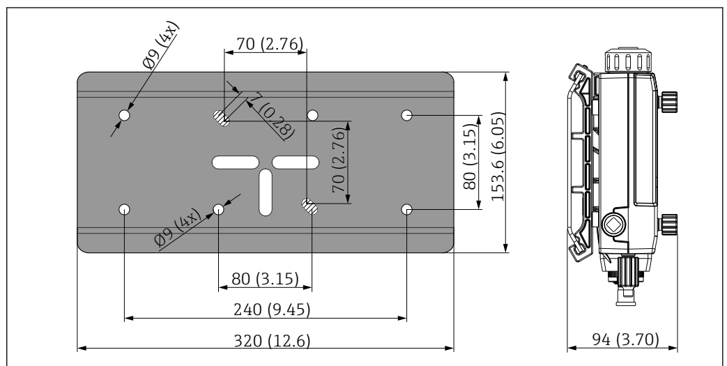
5 Dimensioni del supporto da parete. Unità ingegneristica: mm (in)
