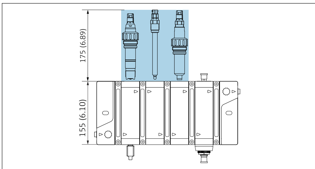
2 Distanza di montaggio. Unità ingegneristica: mm (in)
