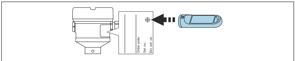
31 Test funcțional cu magnet de testare
