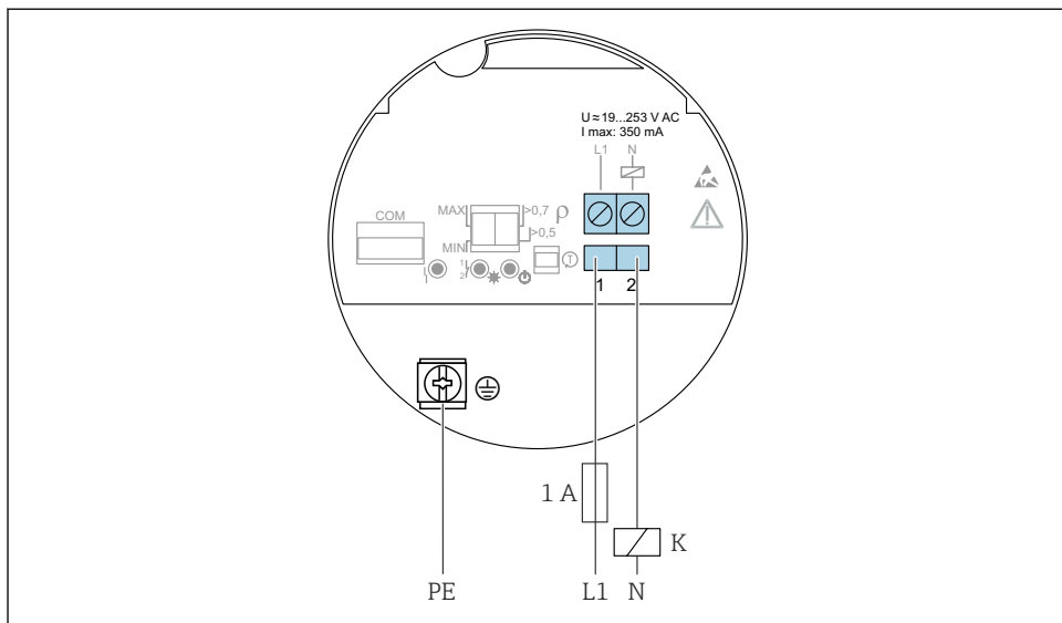
14 2 cabluri c.a., inserție electronică FEL61
