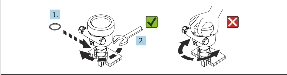
11 Înfiletarea dispozitivului
