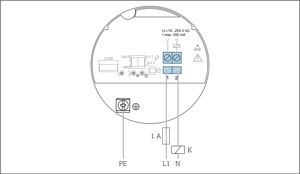
14 AC 2 fils, électronique FEL61
