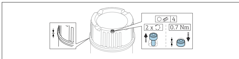
13 Couverture avec vis de fixation
