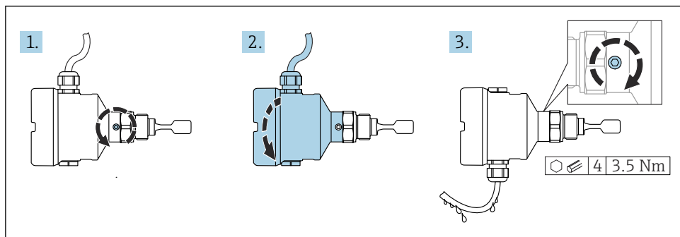
12 Pouzdro s vnějším zajišťovacím šroubem a odkapávací smýčkou
