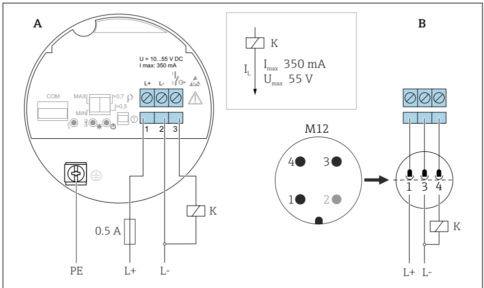
17 Třívodičové provedení DC-PNP, elektronická vložka FEL62
