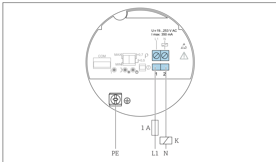
14 2-проводное подключение перем. тока, электронная вставка FEL61
