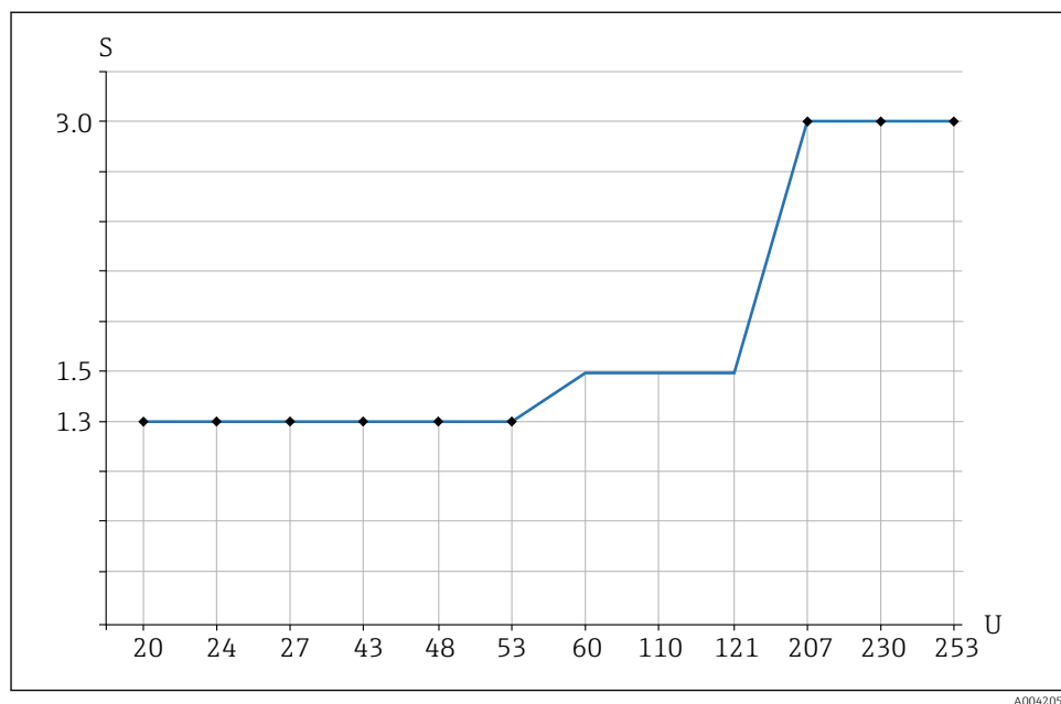
16 Рекомендуемая минимальная удерживающая/номинальная мощность для нагрузки
