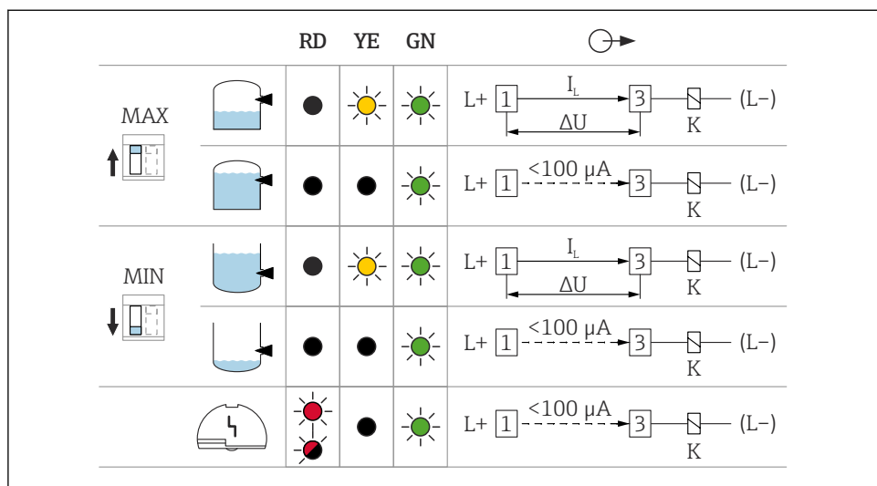
18 Поведение релейного выхода и сигнализации, электронная вставка FEL62
