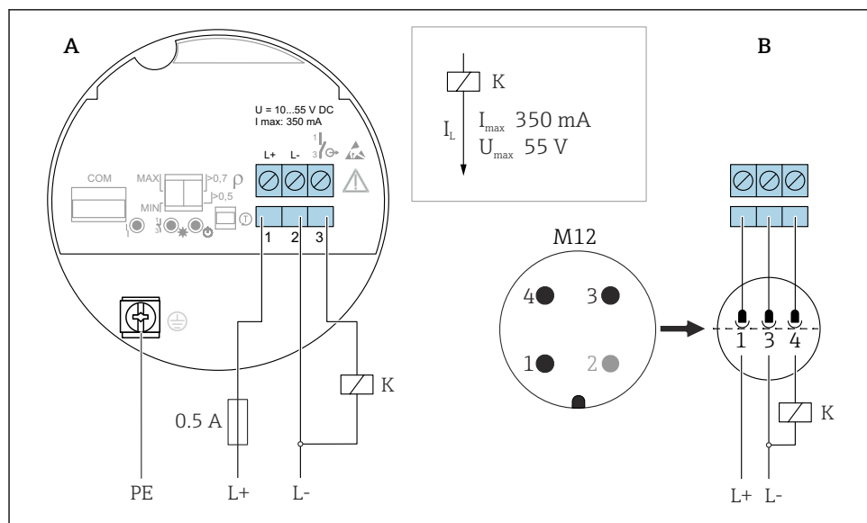
17 3-проводное подключение пост. тока (DC), PNP (электронная вставка FEL62)
