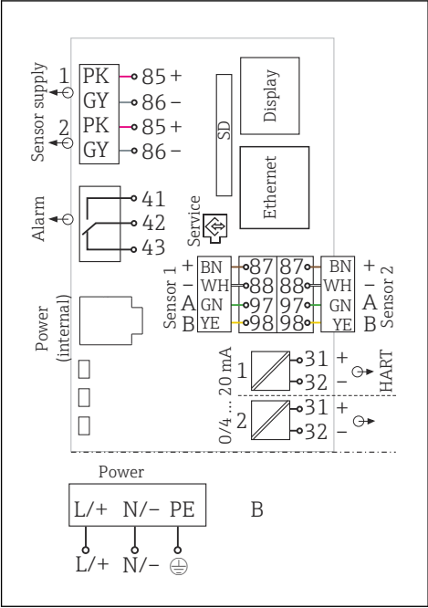
25 Diagrama de conexión completo con el ejemplo del BASE2-E y fuente de alimentación de expansión (B)
