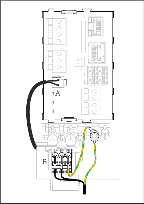
24 Conexión de la fuente de alimentación con el ejemplo del BASE2-E (equipo de campo)
