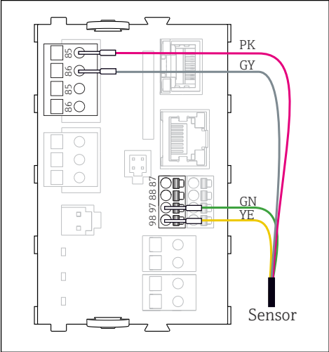
31 Memosens sensores con fuente de alimentación adicional
