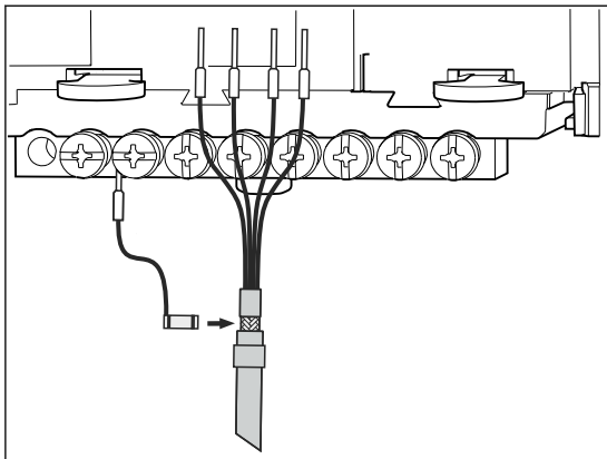
29 Conexión de tierra funcional
