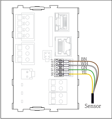
30 Memosens sensores sin fuente de alimentación adicional
