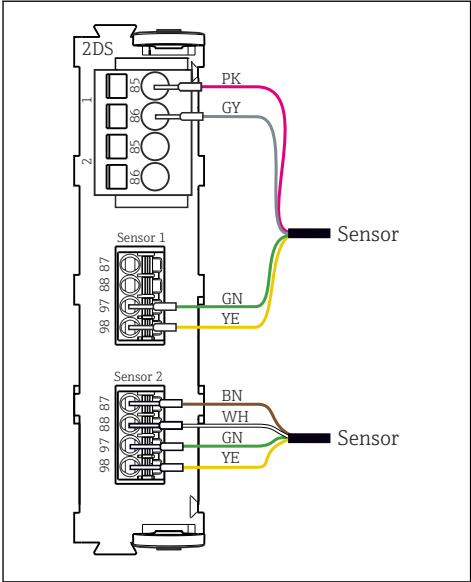
32 Sensores con y sin tensión de alimentación adicional en el módulo del sensor 2DS
