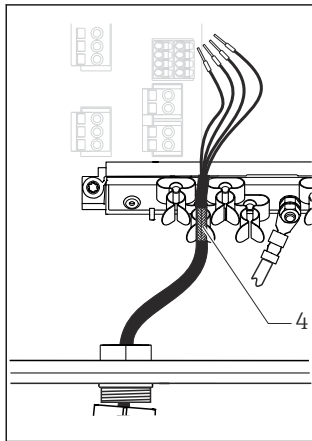
21 Cable con terminación
