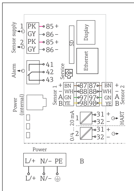
27 Diagrama de conexión completo con el ejemplo del BASE2-E y fuente de alimentación externa (B)
