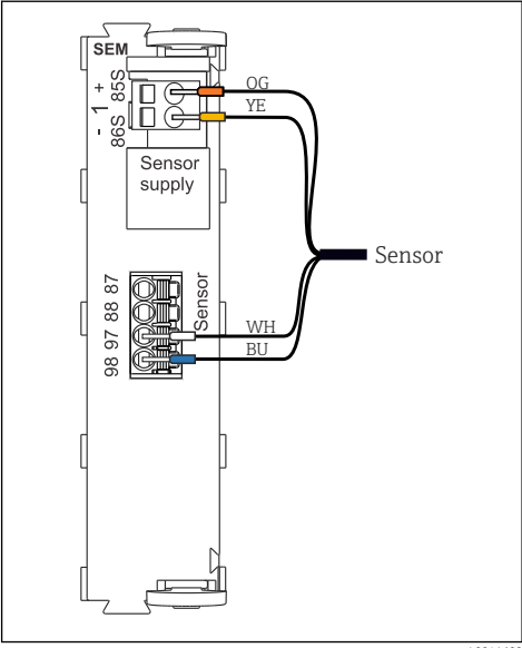
33 Conexión del espectrómetro al módulo SEM
