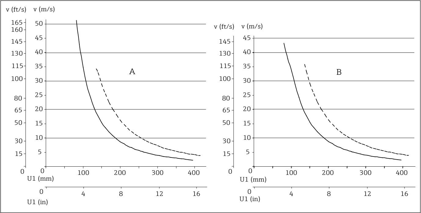
8 Velocità di deflusso consentita in base alla lunghezza di immersione
