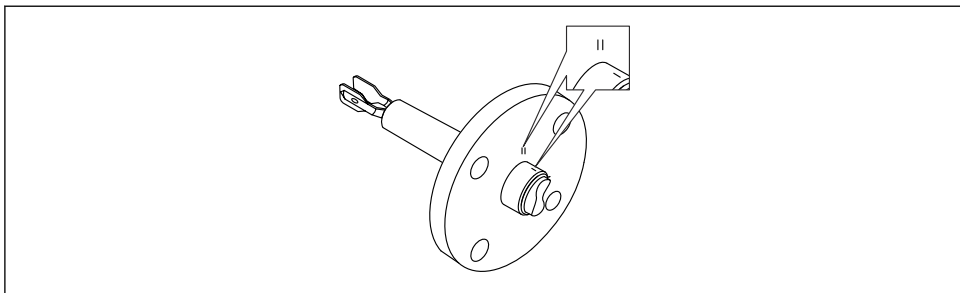
图 8 参照标记水平安装在罐体中时的叉体位置
