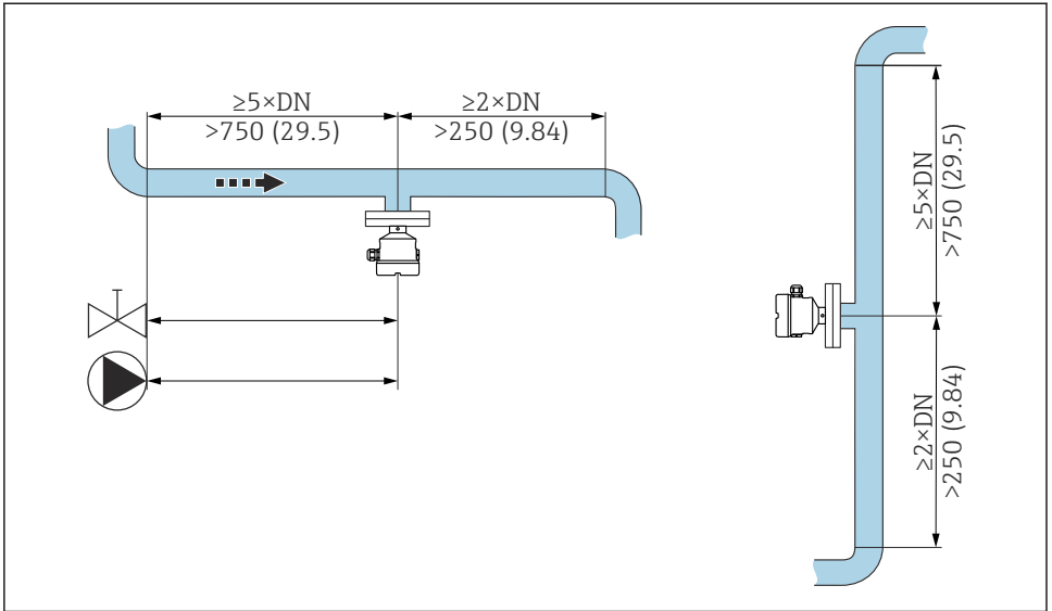
图 4 前直管段的安装。测量单位 mm (in)
