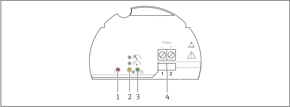
图 15 电子插件 FEL60D
