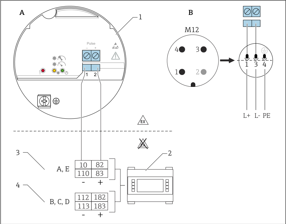
图 12 电子插件 FEL60D 和密度计算仪 FML621 的接线图
