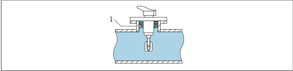
图 2 安装实例：叉体接触管道内流动的介质
