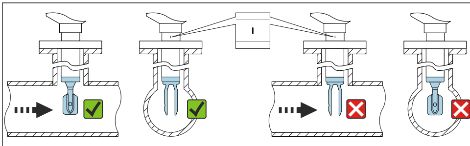
图 9 安装在管道中（注意叉体安装位置和标记）
