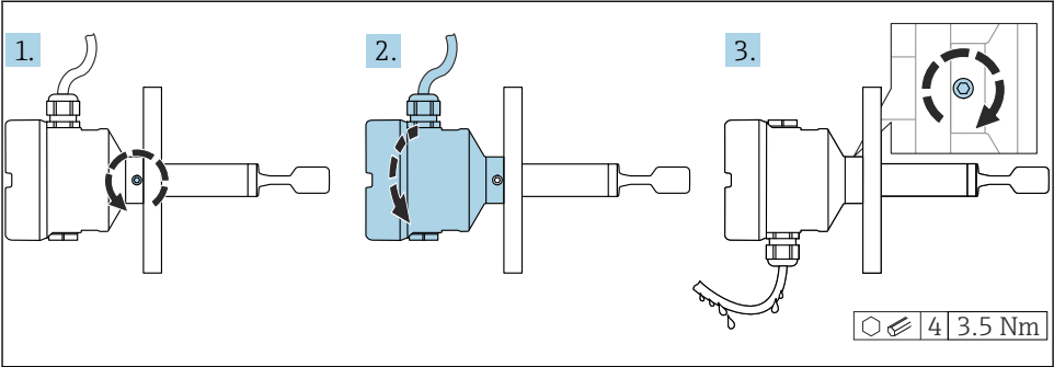
图 10 外壳带外部锁紧螺丝和排水回路
