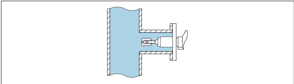
图 3 安装实例：叉体不接触管道内流动的介质
