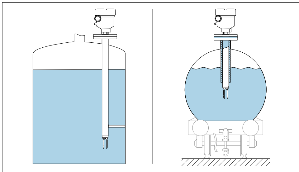
图 7 存在动态负载时，应支撑仪表
