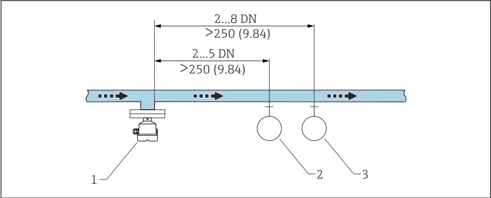
图 5 后直管段的安装。测量单位 mm (in)
