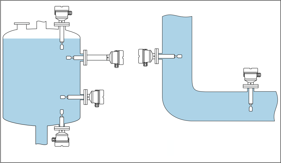
1 安装实例：安装在容器、罐体或管道中
