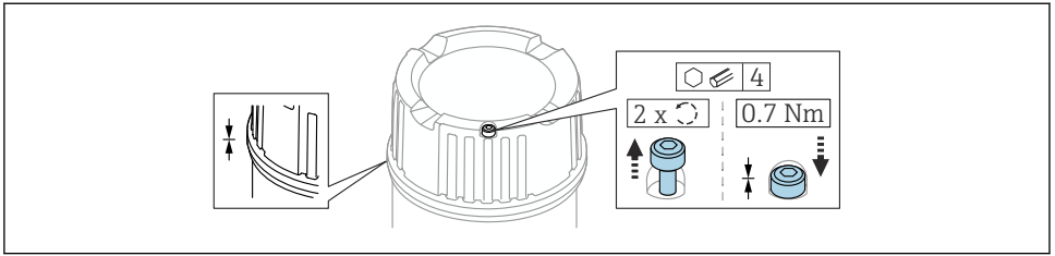
图 11 带锁定螺丝的外壳盖
