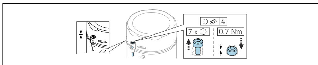
6 Крышка с крепежным винтом; гигиеничный корпус (только для пылевзрывозащиты)
