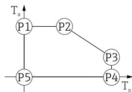
▣ 24 Пластмассовый корпус; рабочая температура 0 до +80 °C ( +32 до +176 °F) для приборов с сертификатом CSA C/US
