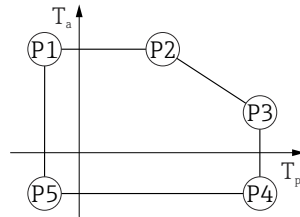
▣ 23 Пластмассовый корпус; рабочая температура -40 до +80 °C ( -40 до +176 °F)
