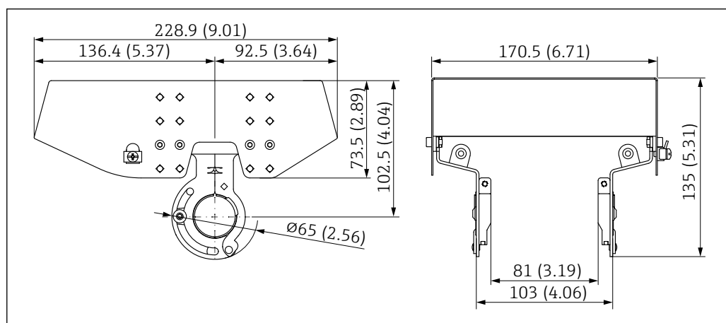
21 Размеры. Единица измерения мм (дюйм)
