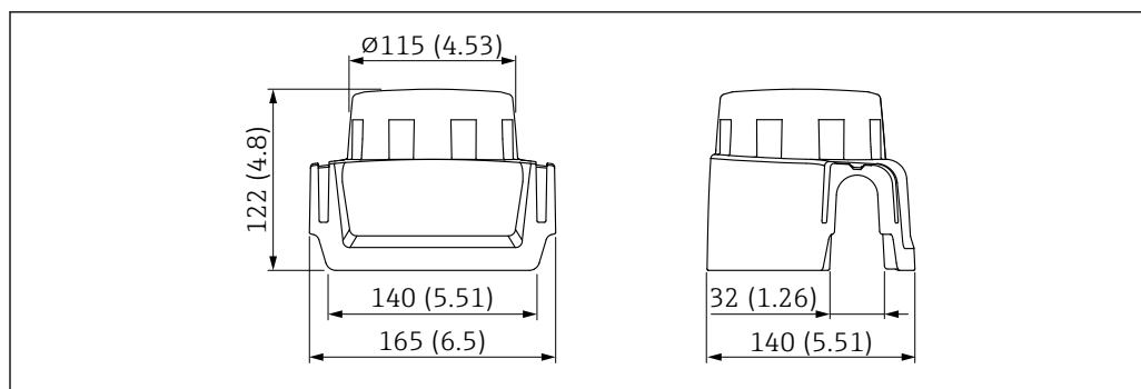
22 Размеры. Единица измерения мм (дюйм)
