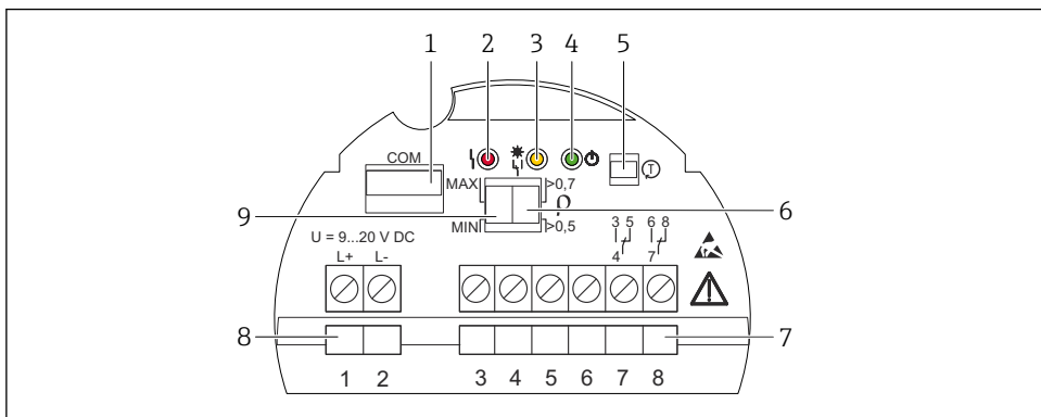
27 Exempel på elektronikinsats FEL64DC
