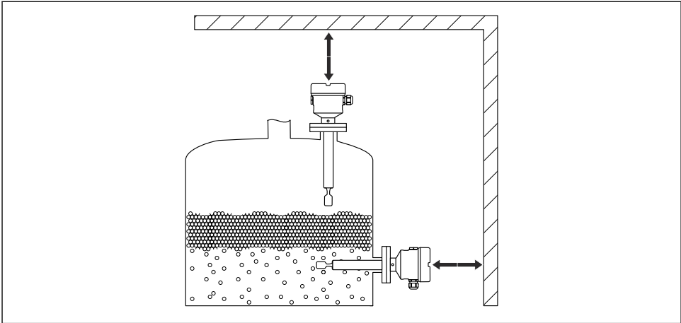
7 Ta med avståndet utanför tanken i beräkningen
