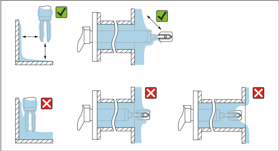
6 Installationsexempel för ett mycket visköst processmedium
