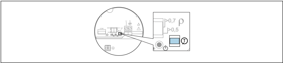
30 Funktionstestknappens placering på elektronikinsatserna FEL61/62/64/64DC/67/68
