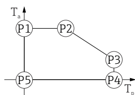
■ 25 Boîtier plastique ; température de process 0 ... +450 °C (+32 ... +842 °F) avec agrément CSA C/US
