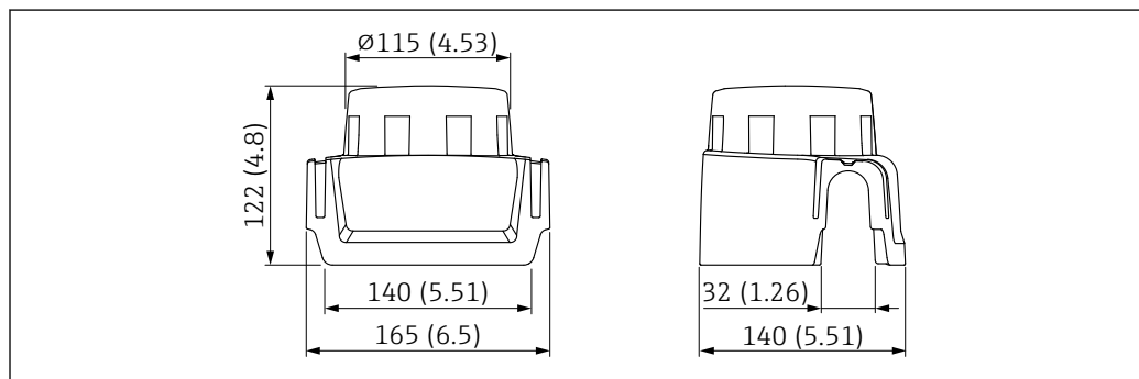
68 Dimensions. Unité de mesure mm (in)
