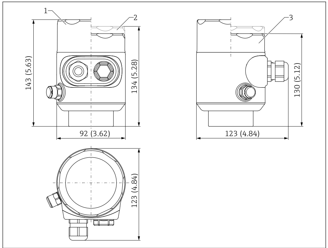
54 Dimensions du boîtier à simple compartiment 316L, app. hygiénique. Unité de mesure mm (in)
