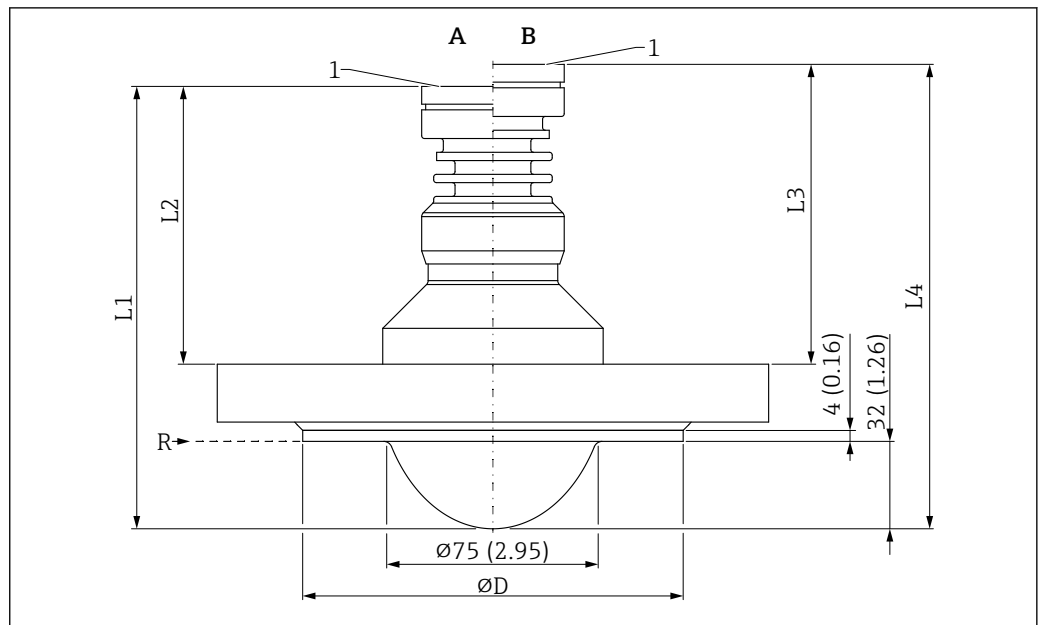
60 Dimensions de l'antenne, plaquée PTFE, affleurante, 80 mm (3 in), avec bride. Unité de mesure mm (in)
