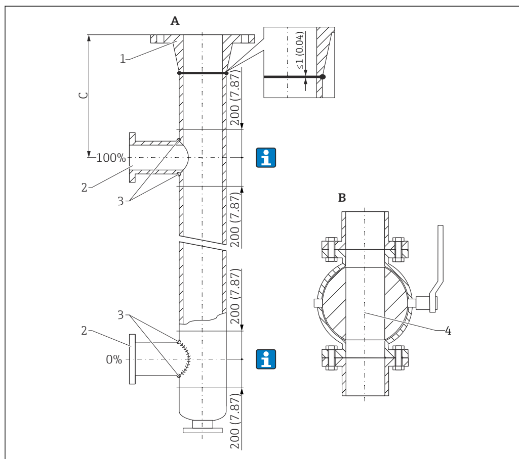
13 Exemple de construction de bypass. Unité de mesure mm (in)
