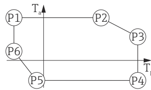
28 Boîtier plastique ; température de process -196 \dots +200 \text{ }^{\circ}\text{C} ( -320 \dots +392 \text{ }^{\circ}\text{F} )
