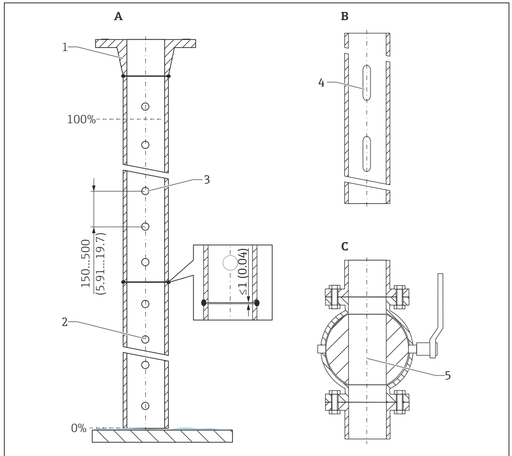
11 Exemple de construction de tube de mesure. Unité de mesure mm (in)
