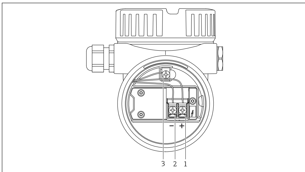
■ 6 Bornes de raccordement et borne de terre dans le compartiment de raccordement
