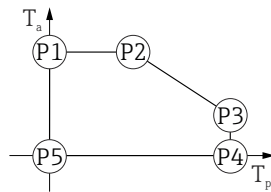
29 Agrément CSA C/US and boîtier plastique ; température de process 0 \dots +200 \text{ }^{\circ}\text{C} ( +32 \dots +392 \text{ }^{\circ}\text{F} )
