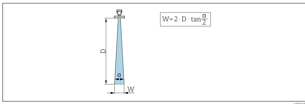
9 Relation entre l'angle d'émission \alpha , la distance D et la largeur de faisceau W
