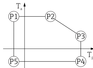
30 Boîtier alu, revêtu ; température de process -20 \dots +150 \text{ }^{\circ}\text{C} ( -4 \dots +302 \text{ }^{\circ}\text{F} )
