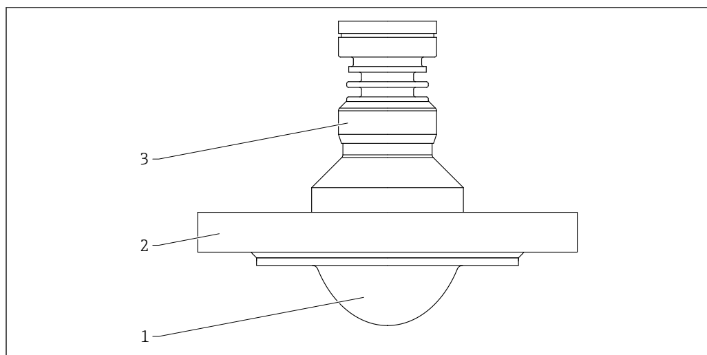
64 Matériau ; antenne, plaquée PTFE, affleurante, 80 mm (3 in), avec bride
