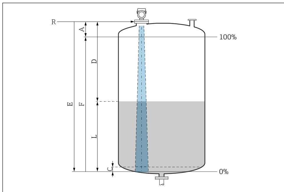
6 Configuratieparameters voor niveaumeting in vloeistof
