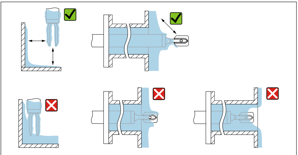
▣ 5 Primjeri instalacije za visoko viskozni procesni medij
