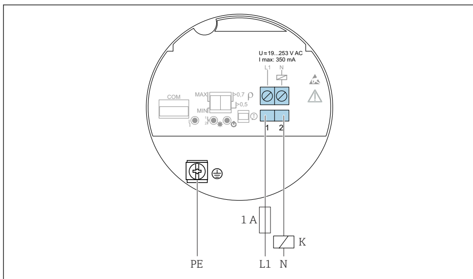
13 2-trådsledning, växelström, elektronikinsats FEL61
