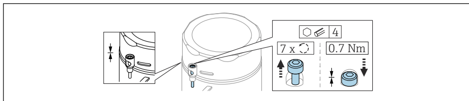
2 Deksel met borgschroef; hygiënische behuizing (alleen voor stofexplosieveiligheid)
