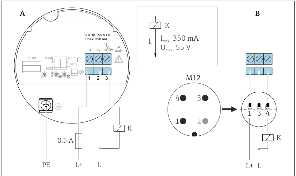
19 3-tråds likströms-PNP, likström, elektronikinsats FEL62
