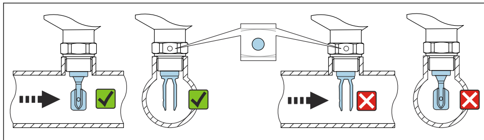
10 Ugradnja u cijevima (uzmite u obzir položaj vilice i oznake)
