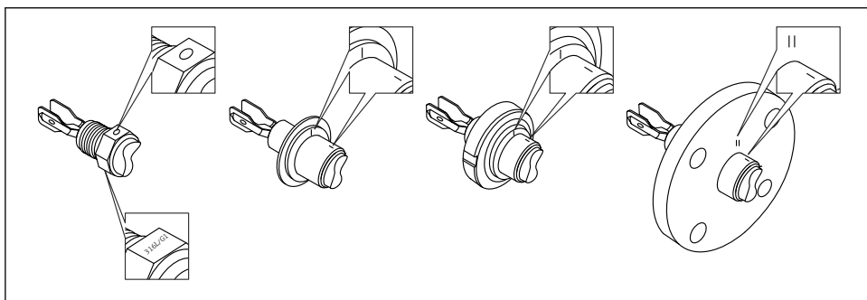
9 Položaj vilice za prilagođavanje kad je postavljena vodoravno u spremniku uz pomoć oznake
