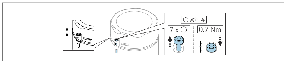
15 Poklopac sa sigurnosnim vijkom; higijensko kućište (samo za zaštitu od zapaljenja prašine)
