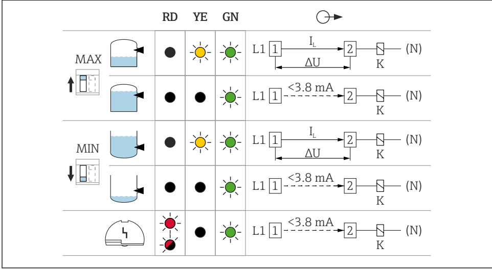
17 Siviç çıkışının davranışı ve sinyaller, elektronik devre FEL61
