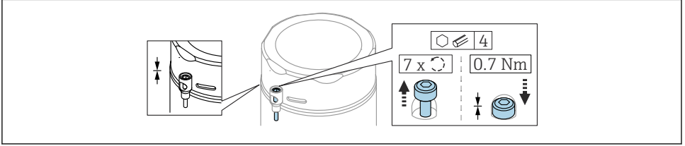
15 Sabitleme vidalı kapak; hijyenik muhafaza (sadece toz patlamasına karşı koruma için)
