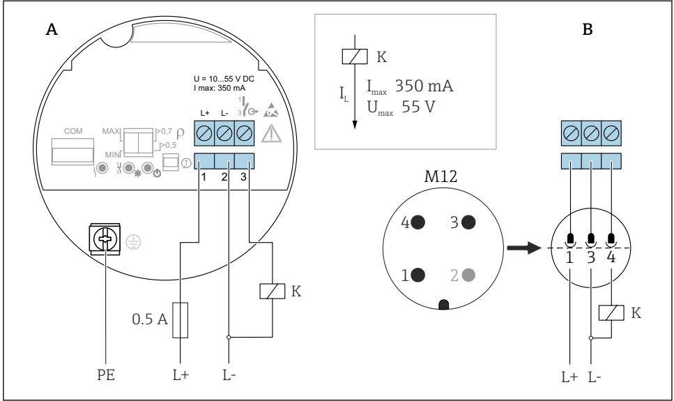
19 3 telli DC-PNP, elektronik parça FEL62
