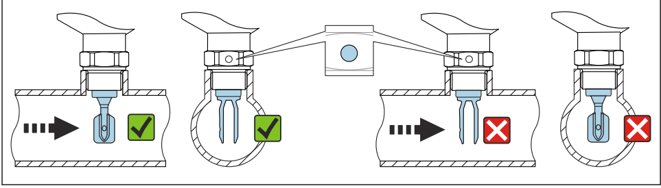
10 Boruya kurulum (çatal pozisyonunu ve işareti dikkate alın)
