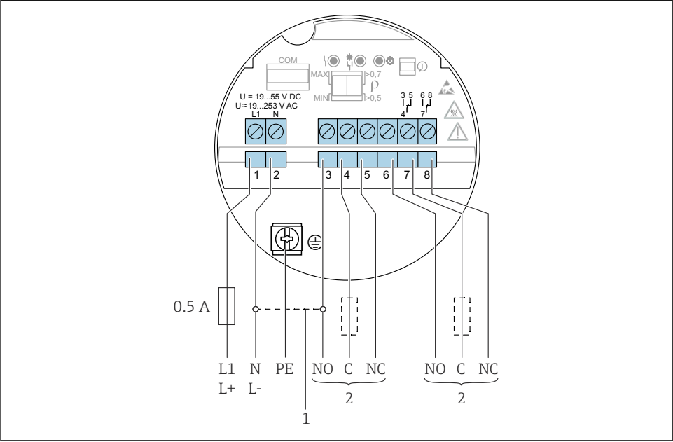
21 Rôle çıkışlı üniversal akım bağlantısı, elektronik devre FEL64
