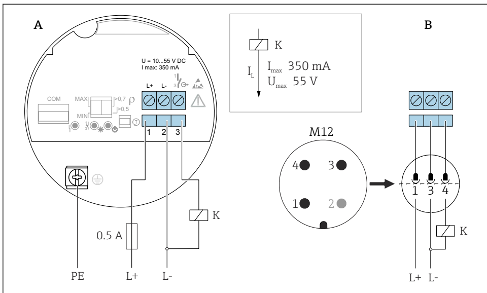
19 3-žična povezava, enosmerna napetost DC, preklapljanje PNP, elektronski vložek FEL62
