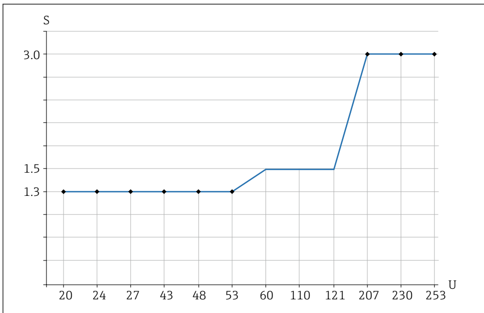
18 Priporočena najmanjša navidezna moč/nazivna moč za breme
