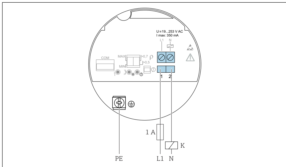
16 2-žična povezava, izmenična napetost "AC", elektronski vložek FEL61
