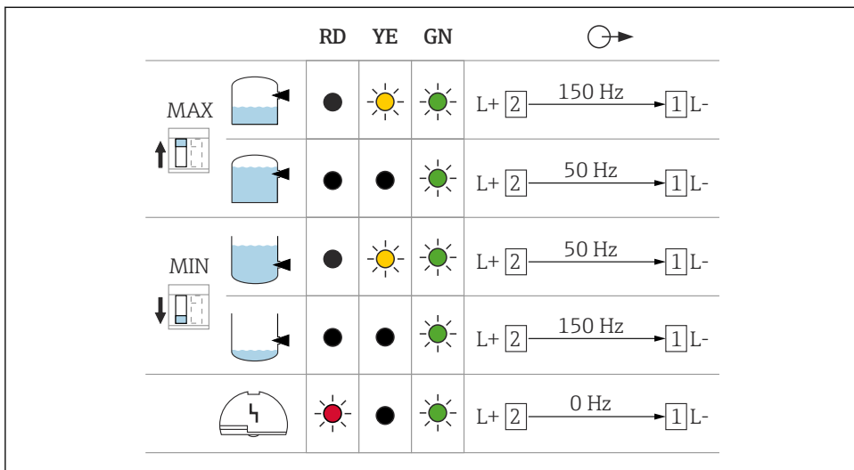
▣ 26 Preklopno vedenje in signalizacija, elektronski vložek FEL67
