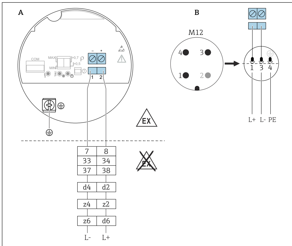
▣ 25 PFM izhod, elektronski vložek FEL67
