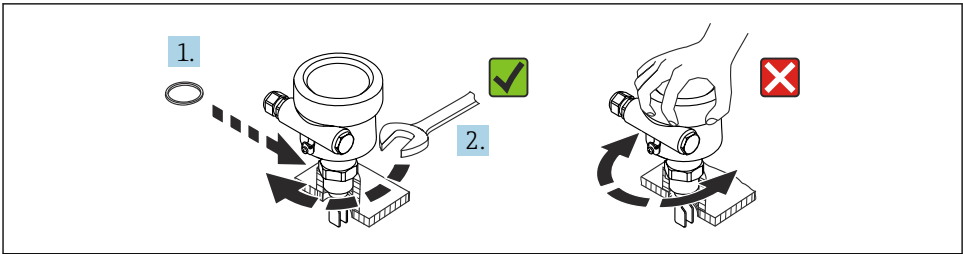
11 Privijanje naprave
