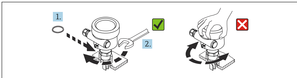
11 Instrument inschroeven
