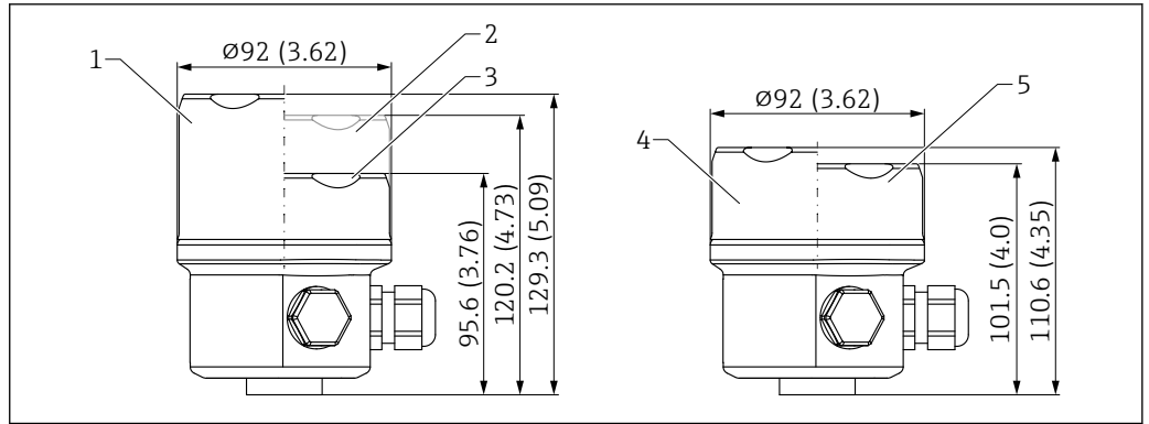
34 Dimensions du boîtier à simple compartiment, 316L, hygiénique. Unité de mesure mm (in)
