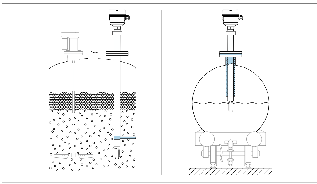
27 Exemples de support en cas de charge dynamique
