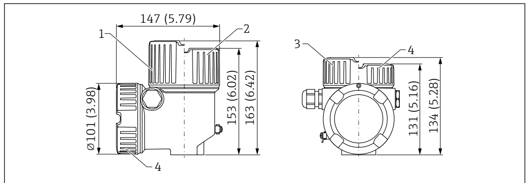
35 Dimensions du boîtier à double compartiment, en forme de L, aluminium, revêtu ; également avec Ex d/XP, Ex "poussières". Unité de mesure mm (in)
