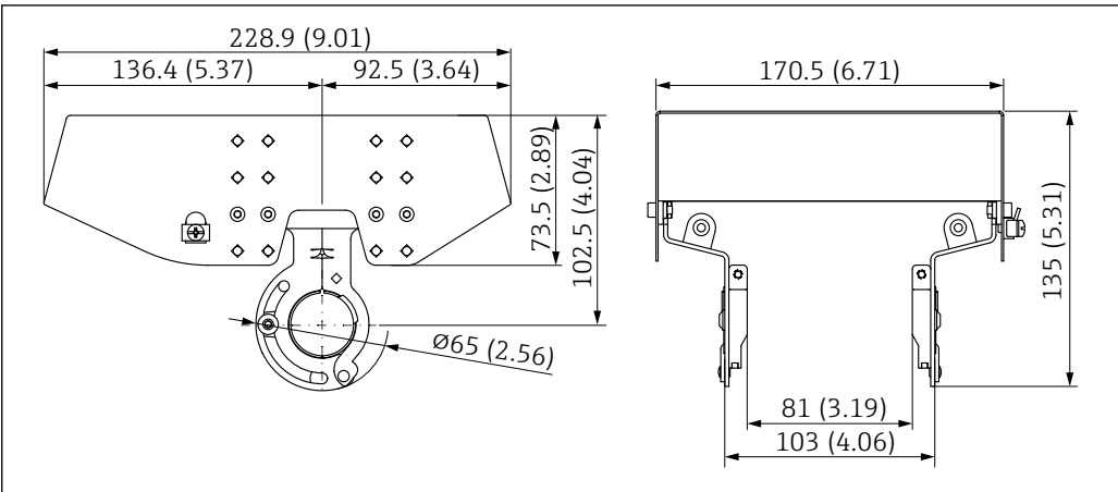
55 Capot de protection pour boîtier à double compartiment en aluminium. Unité de mesure mm (in)
