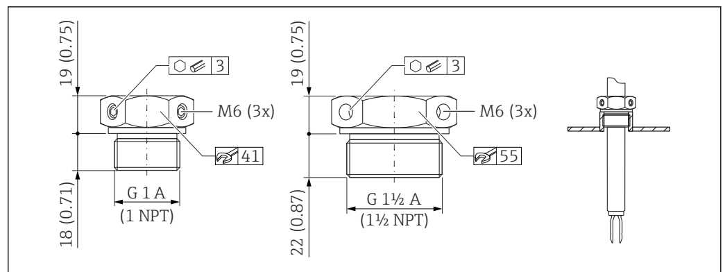
59 Manchons coulissants pour un fonctionnement sans pression p_e = 0 bar (0 psi). Unité de mesure mm (in)
