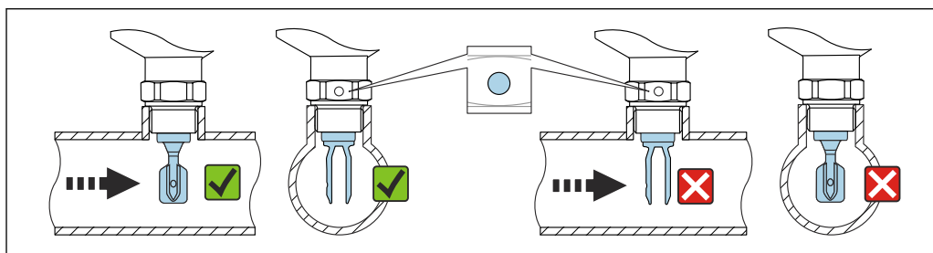
24 Montage dans des conduites (tenir compte de la position de la fourche et du marquage)
