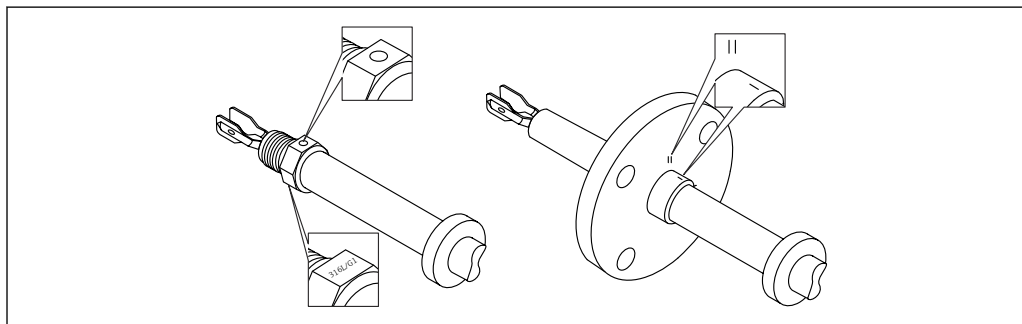
23 Position de la fourche vibrante en cas de montage horizontal dans la cuve à l'aide du repère
