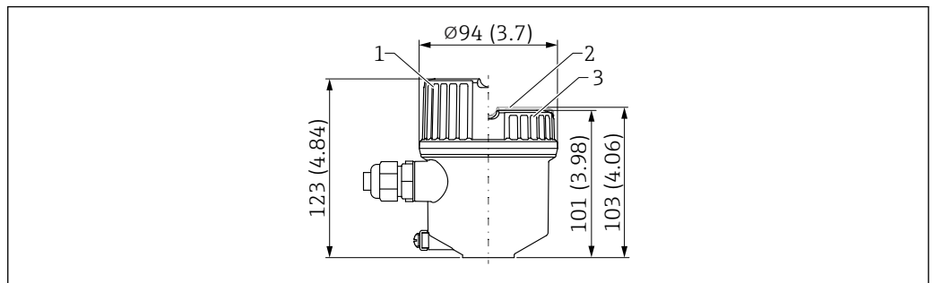
30 Dimensions du boîtier à simple compartiment, plastique. Unité de mesure mm (in)
