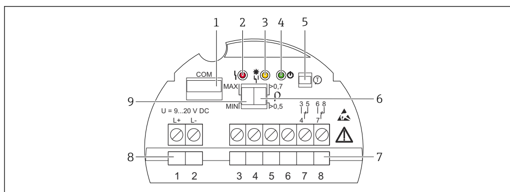
48 Exemple d'électronique FEL64DC
