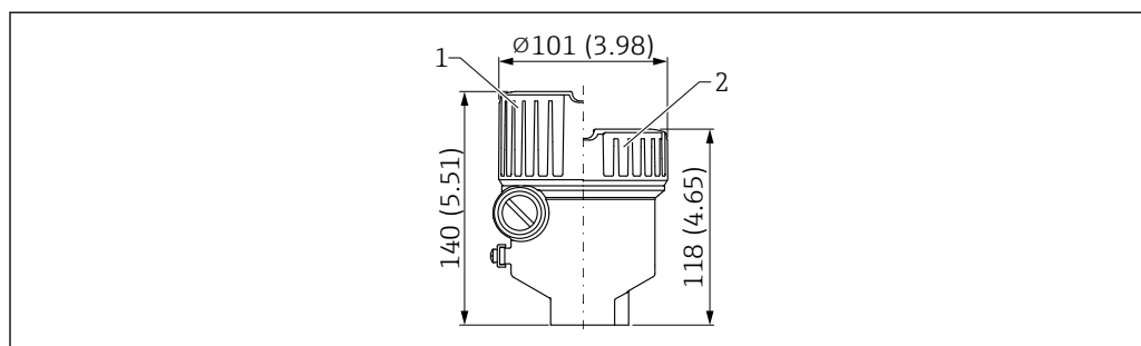
32 Dimensions du boîtier à simple compartiment, aluminium, revêtu ; avec Ex d/XP, Ex "poussières". Unité de mesure mm (in)
