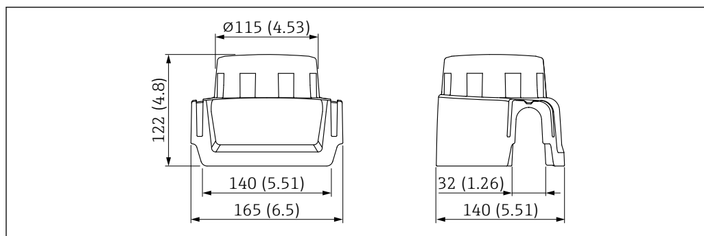
56 Capot de protection pour boîtier à compartiment unique, aluminium ou 316L. Unité de mesure mm (in)
