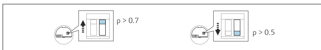
50 Position du commutateur sur l'électronique pour la masse volumique
