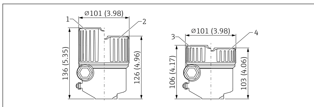
31 Dimensions du boîtier à simple compartiment, aluminium, revêtu. Unité de mesure mm (in)
