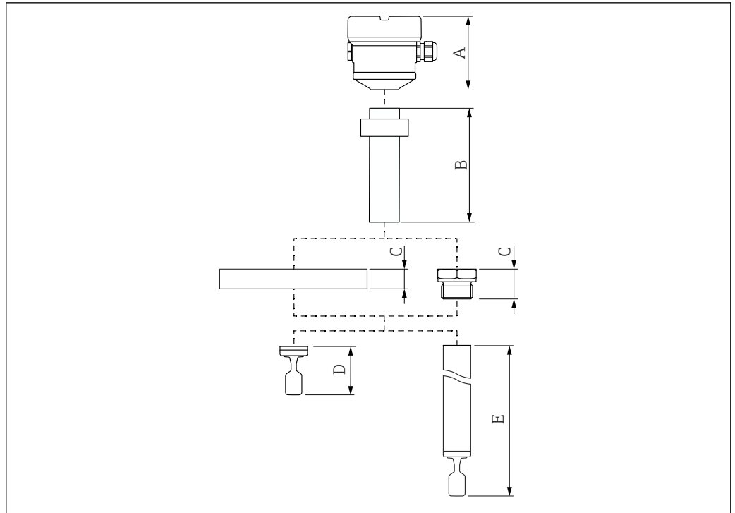
29 Composants permettant de déterminer la hauteur de l'appareil
