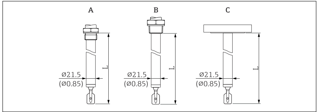
38 Tube prolongateur (longueur L du capteur). Unité de mesure mm (in)
