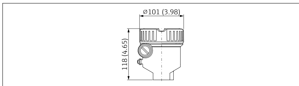
33 Dimensions du boîtier à simple compartiment 316L ; avec Ex d/XP également, Ex "poussières" ; couvercle sans fenêtre. Unité de mesure mm (in)
