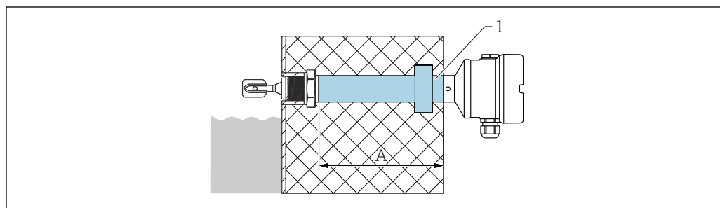
36 Réducteur thermique avec traversée en verre étanche aux gaz
