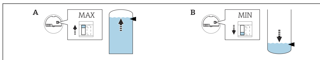
49 Position du commutateur sur l'électronique pour le mode de sécurité MAX/MIN
