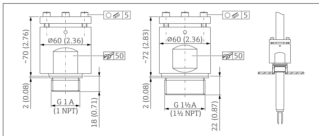
60 Manchons coulissants haute pression. Unité de mesure mm (in)
