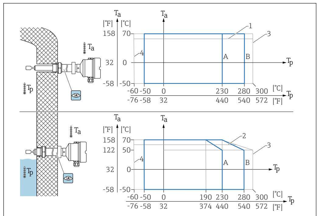
图 28 外壳允许环境温度 T_a 与罐体内部过程温度 T_p 的关系
