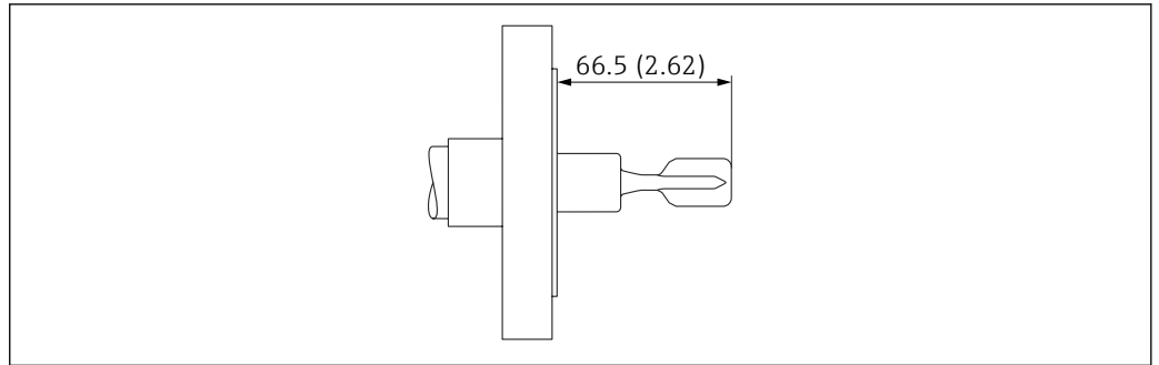
47 法兰连接型传感器示意图。测量单位 mm (in)
