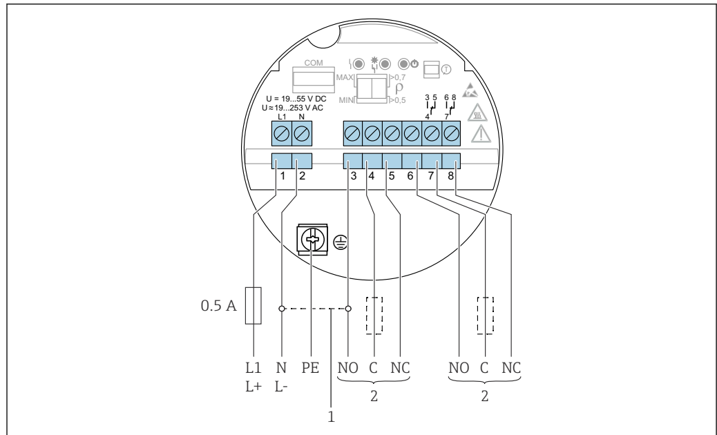
图 7 电子插件 FEL64: 通用电流连接型, 带继电器输出
