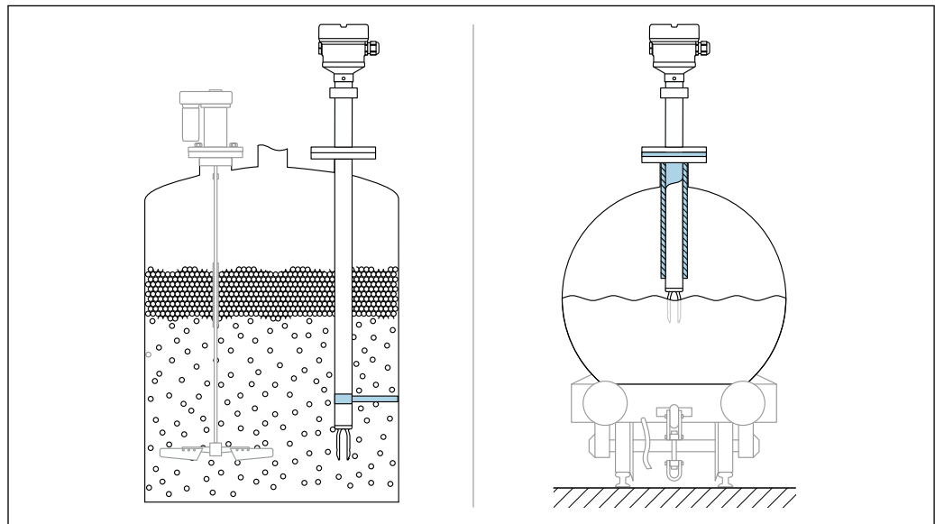
图 27 实例：存在动态负载时，应支撑设备
