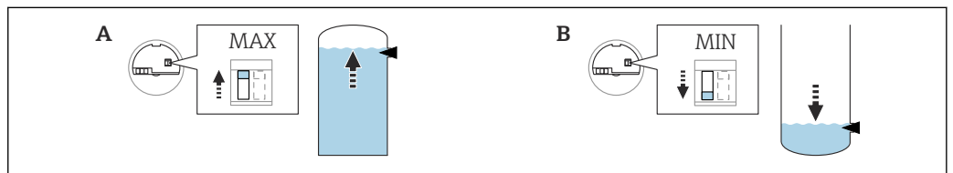
图 49 电子插件上的高限 (MAX) /低限 (MIN) 检测开关位置
