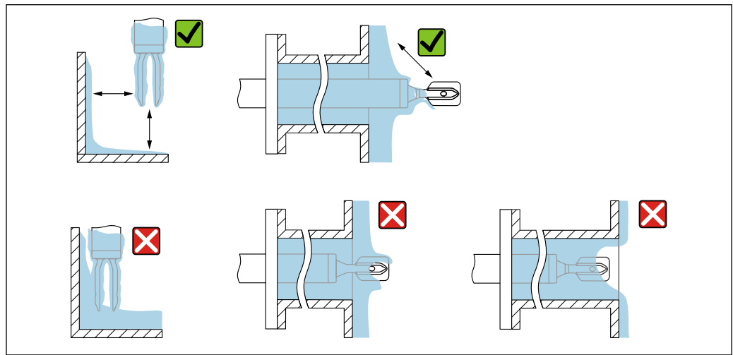
图 21 安装实例：测量高粘度过程介质
