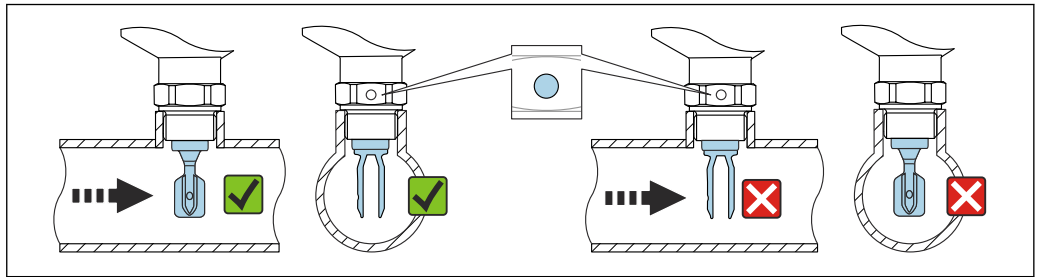
图 24 安装在管道中（注意叉体安装位置和标记）
