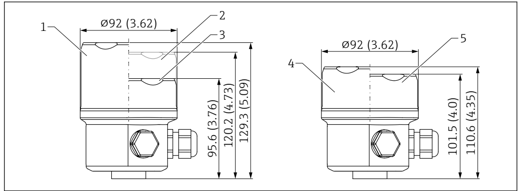
图 34 单腔体 316L 外壳 (卫生型) 的外形尺寸示意图。测量单位 mm (in)
