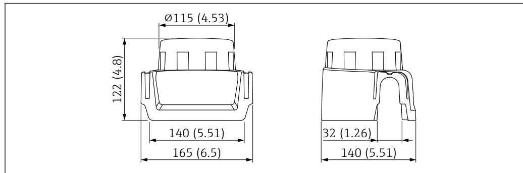
图 56 保护盖, 适用单腔体铝外壳或 316L 外壳。测量单位 mm (in)
