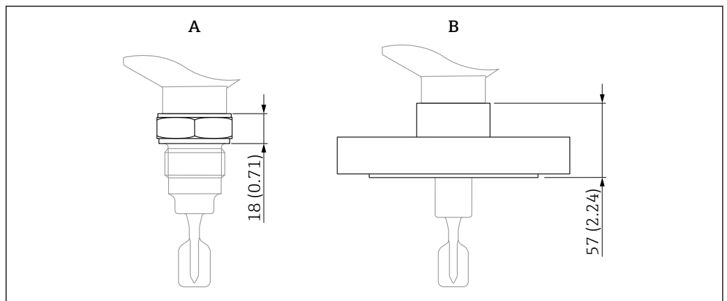
图 40 过程连接的最大高度规格
