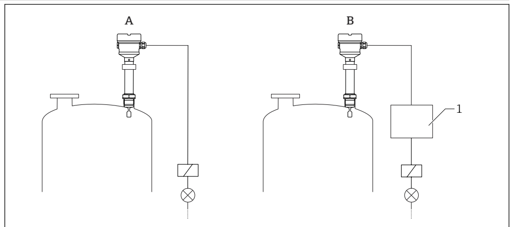
图 1 测量系统示意图
