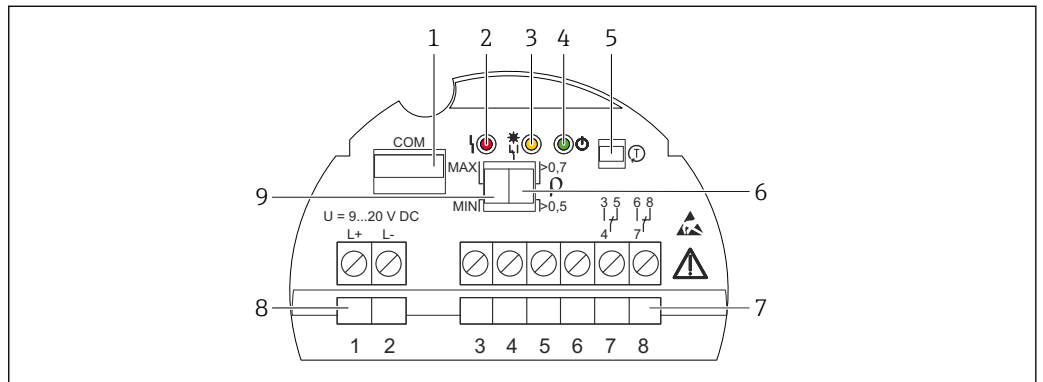
图 48 实例：电子插件 FEL64DC
