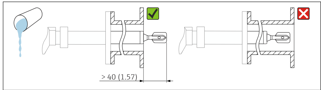
图 20 安装实例：测量高粘度液体。测量单位 mm (in)
