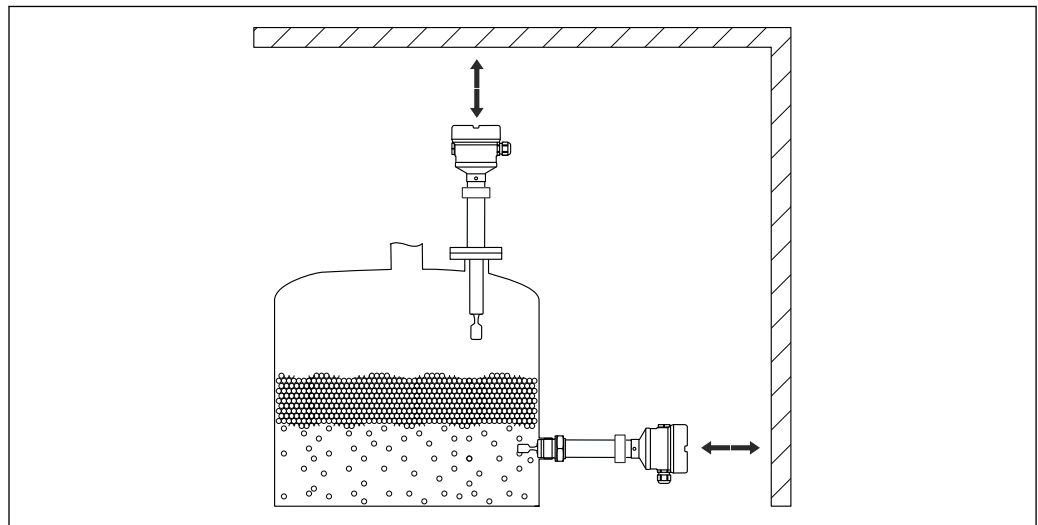
图 22 预留安装间隙
