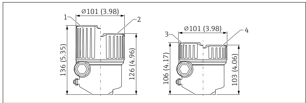
图 31 单腔体铝外壳（带涂层）的外形尺寸示意图。测量单位 mm (in)
