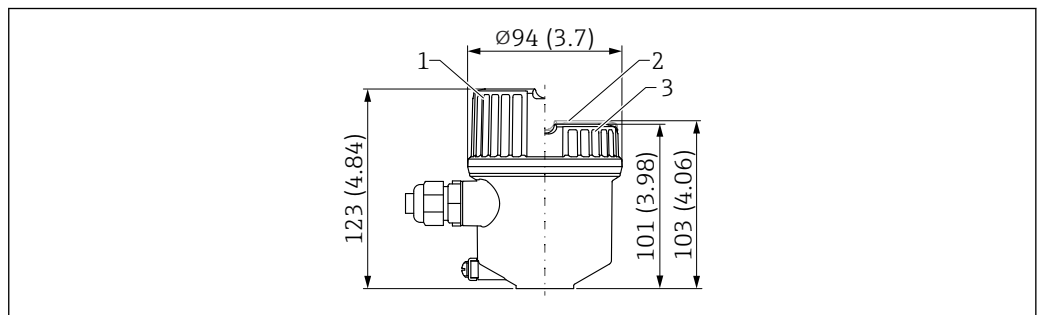
图 30 单腔体塑料外壳的外形尺寸示意图。测量单位 mm (in)
