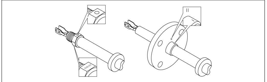
图 23 参照标记水平安装在罐体中时的叉体位置
