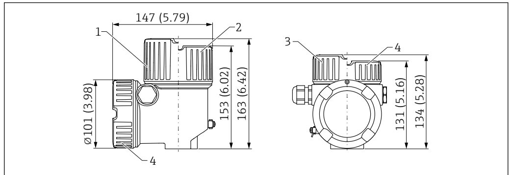
图 35 双腔体 L 型铝外壳 (带涂层) 的外形尺寸示意图; Ex d/XP、粉尘防爆场合。测量单位 mm (in)
