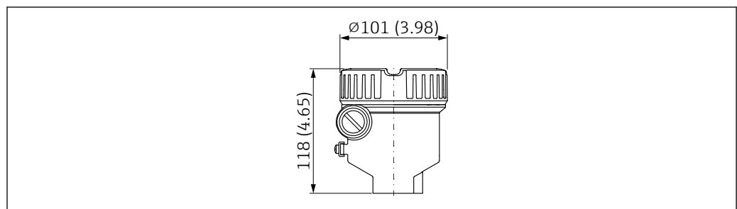
图 33 单腔体 316L 外壳的外形尺寸示意图；Ex d/XP、粉尘防爆场合；外壳盖不带观察窗。测量单位 mm (in)
