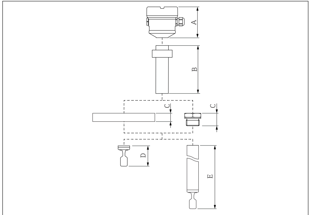
图 29 计算设备高度所需考虑的部件
