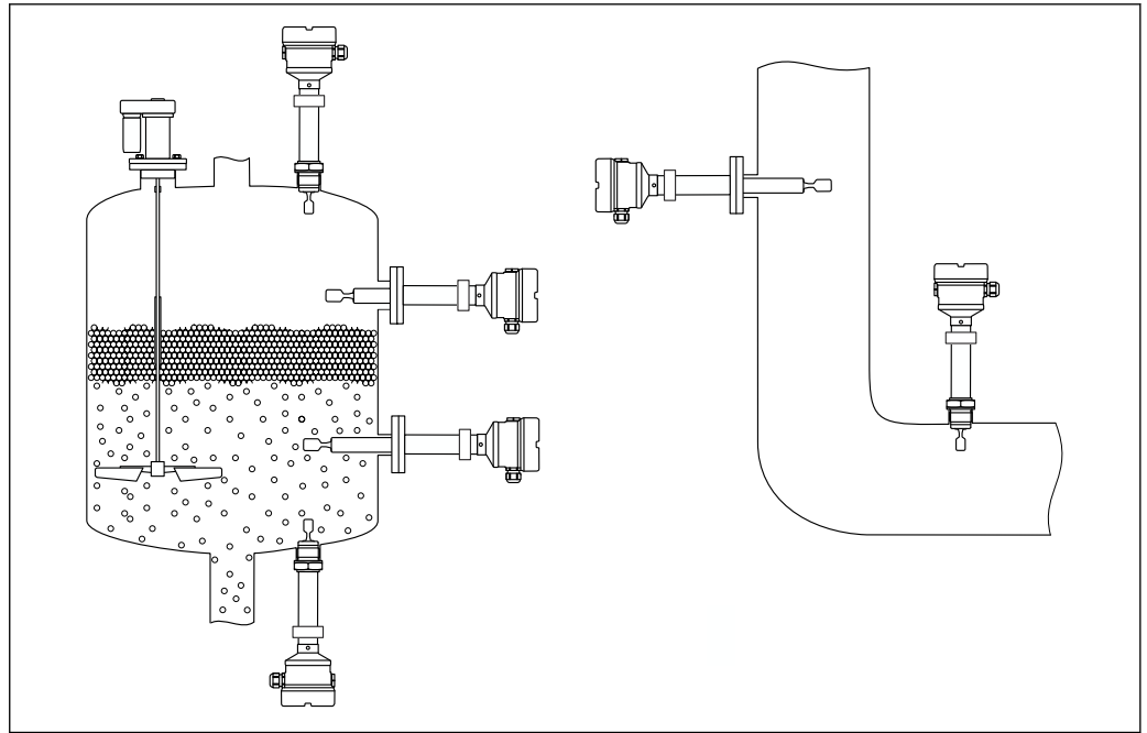
图 18 安装实例：安装在容器、罐体或管道中
