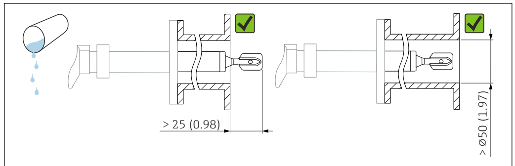
图 19 安装实例：测量低粘度液体。测量单位 mm (in)
