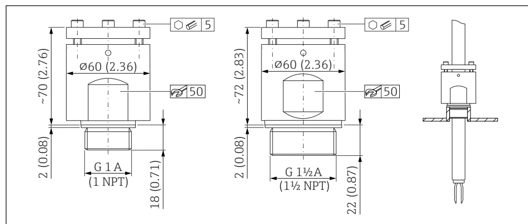
图 60 高压滑动套管。测量单位 mm (in)
