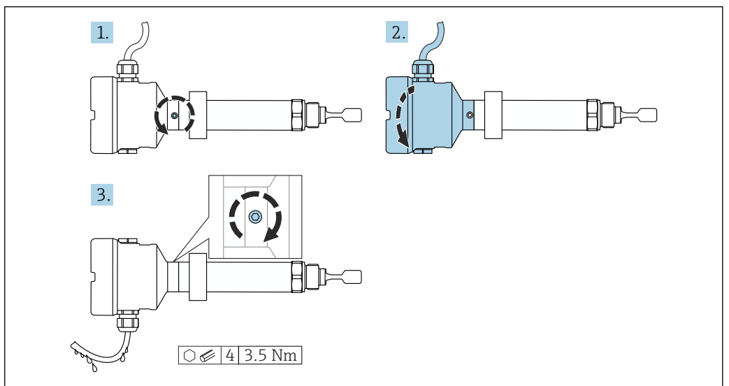
图 25 外壳带外部锁紧螺丝和排水回路
