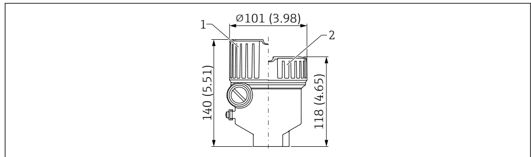
图 32 单腔体铝外壳（带涂层；Ex d/XP、粉尘防爆场合）的外形尺寸示意图。测量单位 mm (in)
