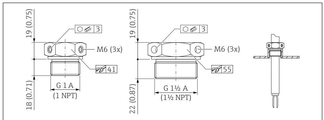
59 常压活动套管 p_e = 0 bar (0 psi)。测量单位 mm (in)
