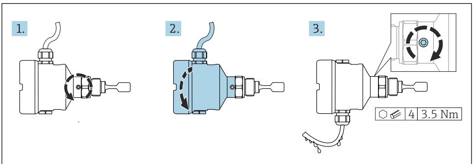
14 Custodia con vite di bloccaggio esterna e anello salvagoccia
