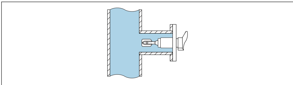
4 Esempio di installazione in tubazioni lontano dal flusso diretto del fluido
