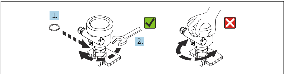
12 Fissaggio del dispositivo
