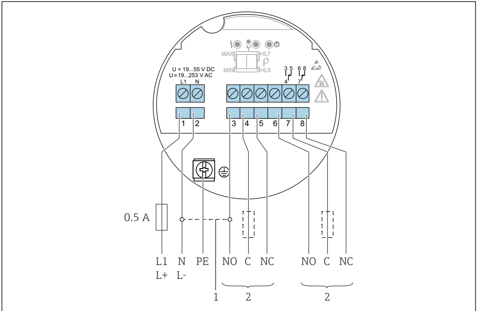
图 16 电子插件 FEL44: 通用电流连接型, 带继电器输出
