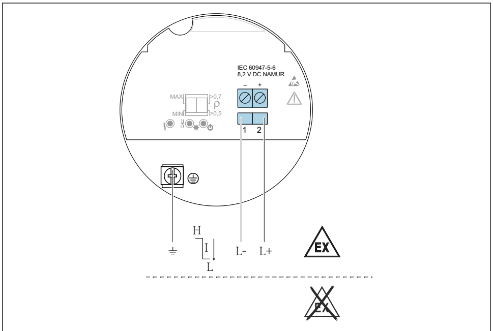
图 18 电子插件 FEL48: 两线制连接, NAMUR 信号 ( \geq 2.2 \text{ mA} / \leq 1.0 \text{ mA} )
