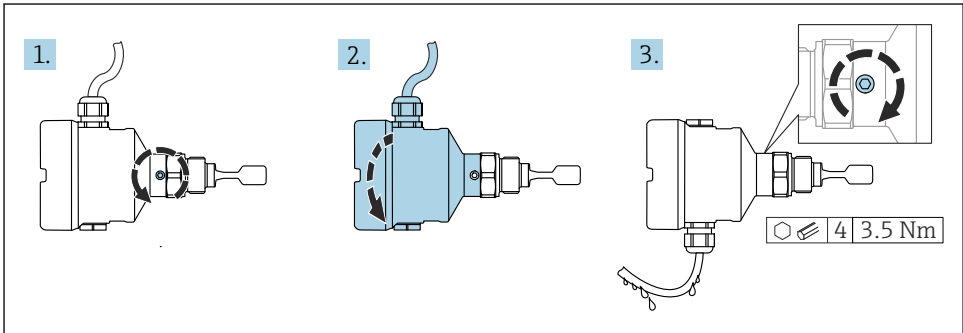
图 12 外壳带外部锁紧螺丝和排水回路
