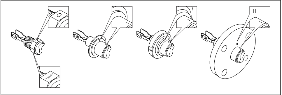
图 9 参照标记水平安装在罐体中的时的叉体位置
