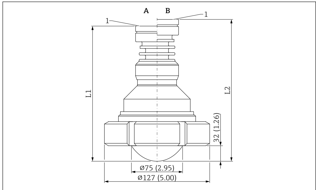
38 Wymiary anteny z pokryciem PTFE, montaż czołowy, 80 mm (3 in), nakrętka rowkowana DIN11851. Jednostka miary mm (in)
