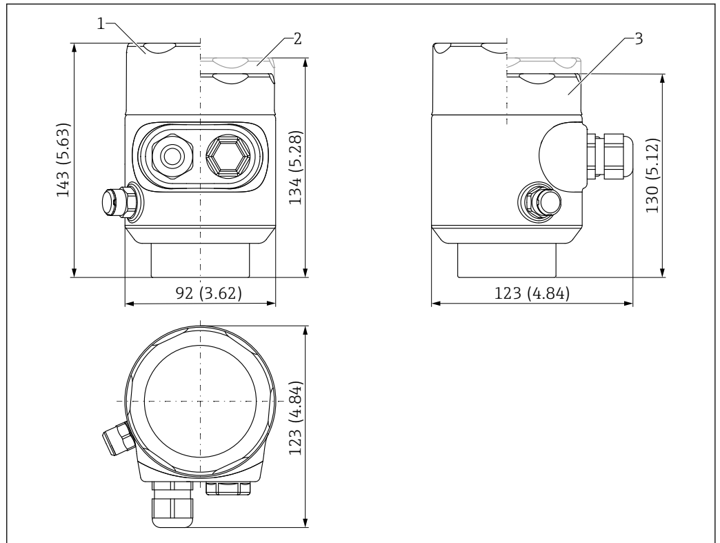
33 Wymiary obudowy jednokomorowej, 316L, wersja higieniczna. Jednostka miary mm (in)
