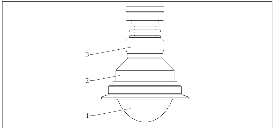
▣ 46 Materiał; antena z pokryciem PTFE, montaż czołowy, 80 mm (3 in), z przyłączem Tri-Clamp ISO2852
