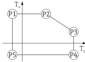
11 Obudowa z tworzywa sztucznego; zakres temperatury medium -20 ... +150 °C (-4 ... +302 °F)
