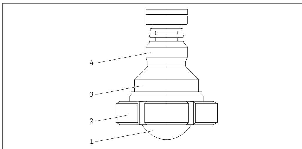
44 Materiał; antena z pokryciem, montaż czołowy, 80 mm (3 in), nakrętka rowkowana DIN11851. Jednostka miary mm (in)
