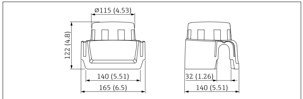
51 Wymiary. Jednostka miary mm (in)
