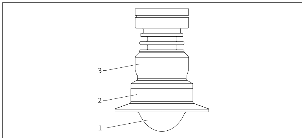
45 Materiał; antena z pokryciem PTFE, montaż czołowy, 50 mm (2 in), z przyłączem Tri-Clamp ISO2852. Jednostka miary mm (in)
