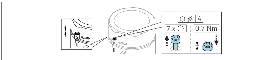
2 Крышка с крепежным винтом; гигиеничный корпус (только для пылевзрывозащиты)
