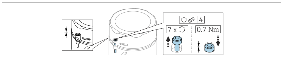
2 Couverture avec vis de sécurité ; boîtier hygiénique (uniquement pour protection Ex poussières)
