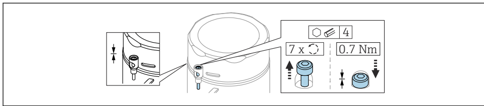
5 Deksel met borgschroef; hygiënische behuizing (alleen voor stofexplosieveiligheid)
