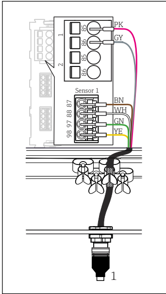
▣ 28 M12 接头（例如在传感器模块上）
