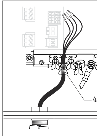
图 17 将电缆连接至接地夹
