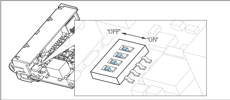
图 55 内部端接的 DIP 开关
