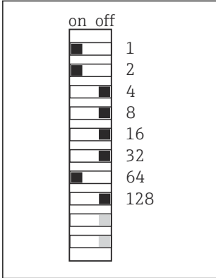
图 57 有效 PROFIBUS 地址 67 图 58 有效 Modbus 地址 195 图 59 无效地址 255 1)
