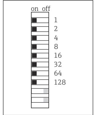
图 57 有效 PROFIBUS 地址 67 图 58 有效 Modbus 地址 195 图 59 无效地址 255 1)
