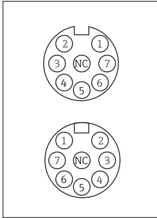
▣ 29 M12 连接头；上图：插座；下图：插头（均为俯视图）
