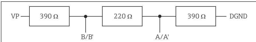
图 56 内部端接示意图
