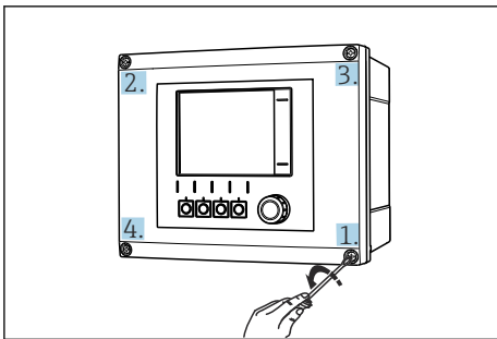
图 13 使用十字螺丝刀沿对角方向依次松开外壳螺丝
