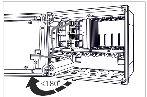
图 14 打开显示单元盖板，最大开度为 180°（取决于安装位置）
