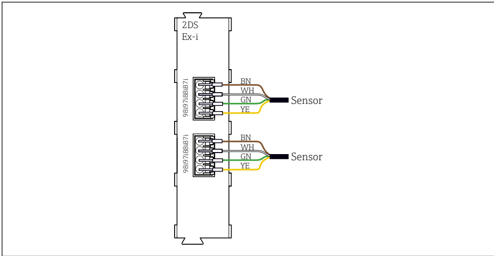
图 30 传感器和本安 Ex-i 型传感器通信模块 2DS，不带附加电源
