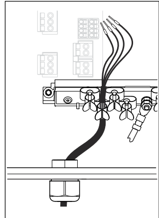
图 18 将电缆安装在接地夹中
