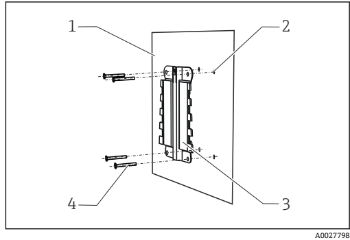
图 10 墙装示意图
