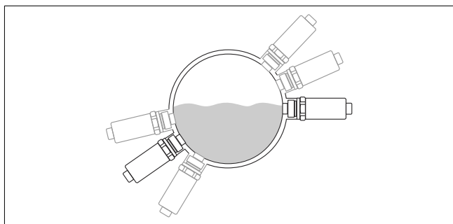
2 Exemples de montage, conduite
