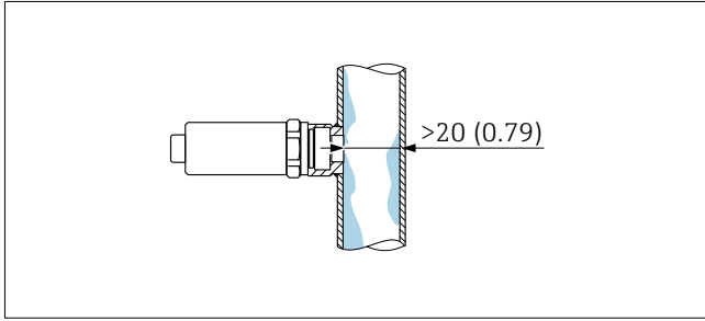
☐ 3 고정성 유체를 위한 플러시 장착 설치, mm (inch) 단위 규격
