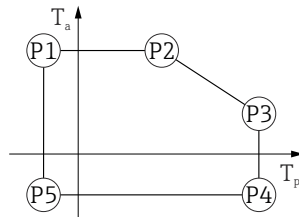
図 9 プラスチックハウジング；プロセス温度 -40～+80 °C (-40～+176 °F)
