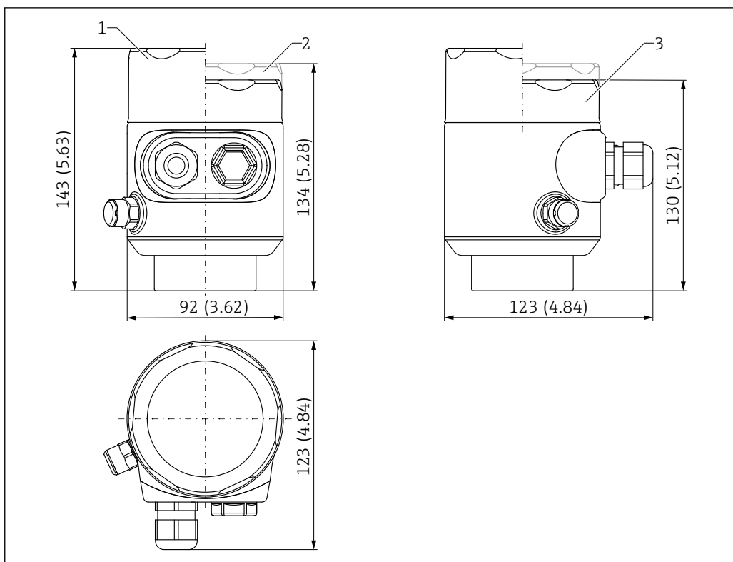
図 21 SUS 316L 相当 シングル端子箱部、サニタリ仕様の寸法。測定単位 mm (in)
