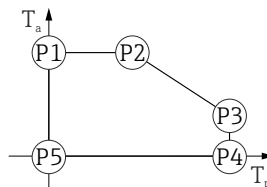
図 10 プラスチックハウジング；プロセス温度 0～+80 °C (+32～+176 °F)、CSA C/US 認定取得
