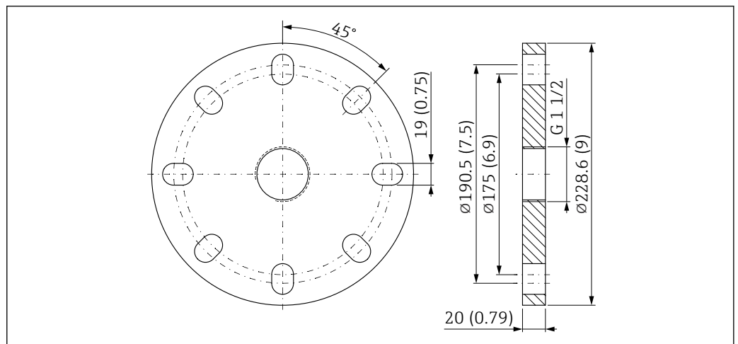
図 32 UNI フランジ 4"/DN100/100A の寸法。測定単位 mm (in)
