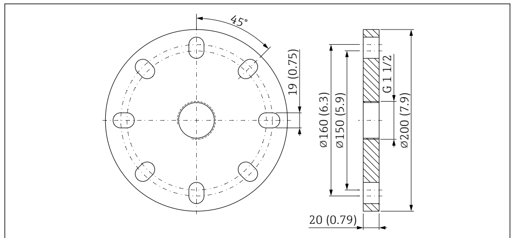
図 31 UNI フランジ 3"/DN80/80A の寸法。測定単位 mm (in)
