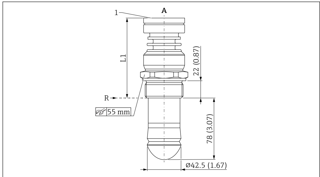
図 29 ドリップオフアンテナ 50 mm (2 in) (ネジ込みプロセス接続) の寸法。測定単位 mm (in)
