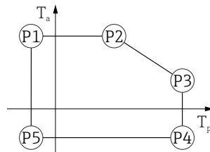
図 18 SUS 316L 相当製ハウジング、サニタリ仕様；プロセス温度 -40\sim+130\text{ }^{\circ}\text{C} ( -40\sim+266\text{ }^{\circ}\text{F} )
