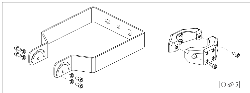
図 42 取付ブラケット（調整可能）の納入範囲
