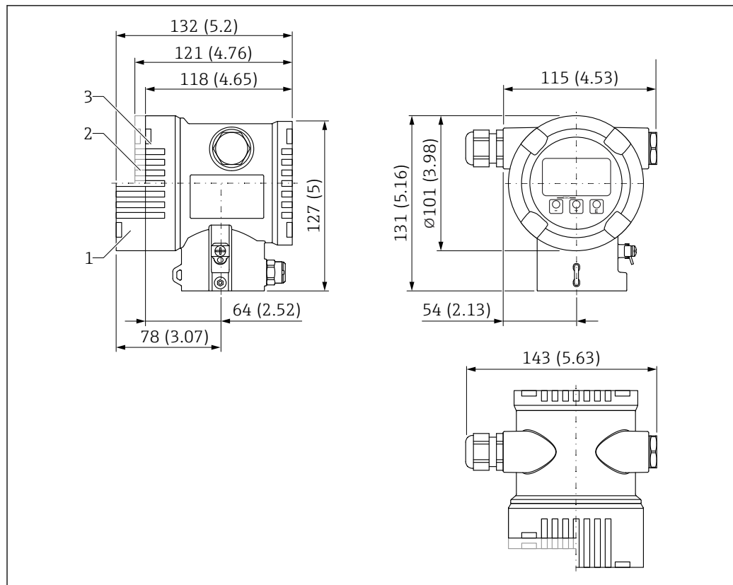
図 22 デュアル端子箱部の寸法。測定単位 mm (in)
