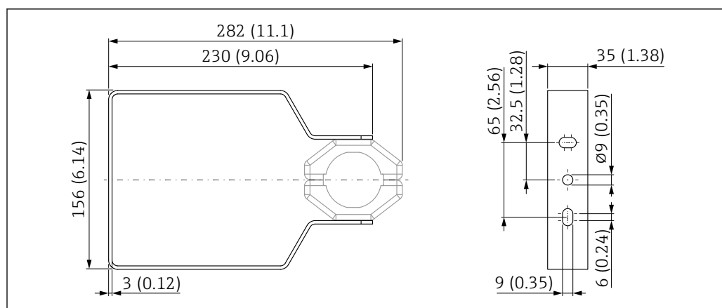
図 41 取付ブラケットの寸法。測定単位 mm (in)
