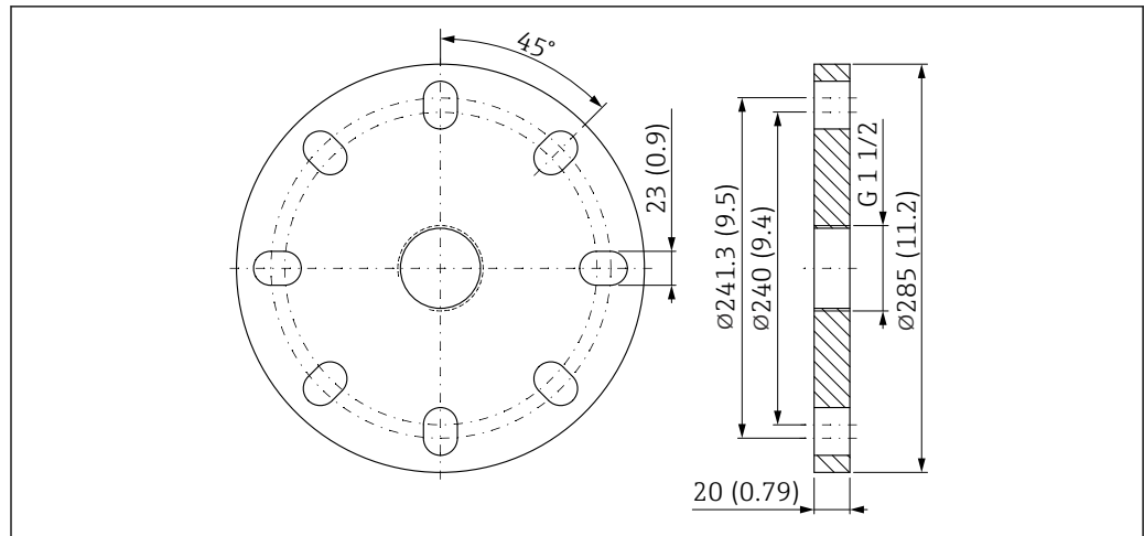
図 33 UNI フランジ 6"/DN150/150A の寸法。測定単位 mm (in)
