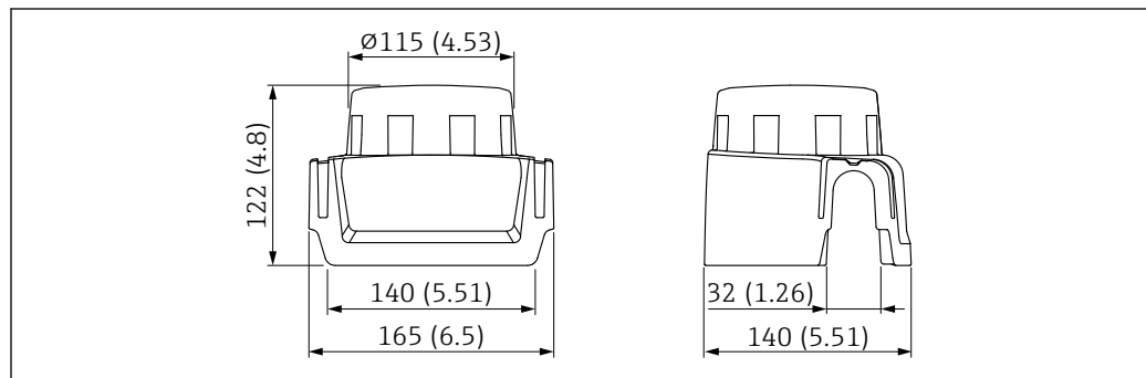
図 39 寸法。測定単位 mm (in)
