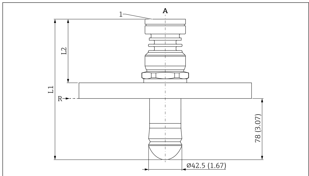
図 30 ドリップオフアンテナ 50 mm (2 in) (UNI フランジプロセス接続) の寸法。測定単位 mm (in)
