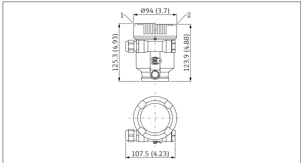
図 19 シングル端子箱部、プラスチック (PBT) の寸法。測定単位 mm (in)
