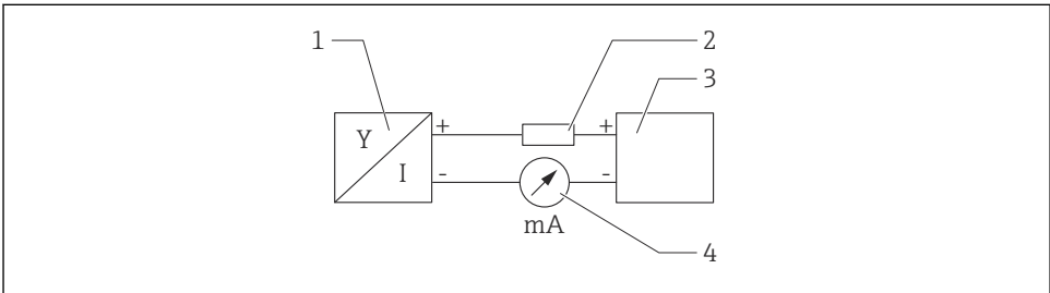
i 15 Blockdiagram över HART-anlutningen
